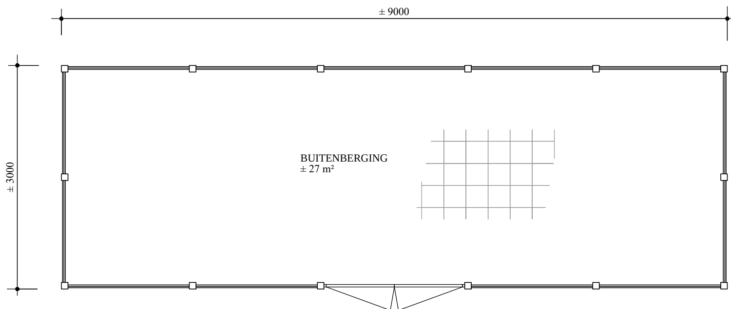
- PLATTE GROND -
