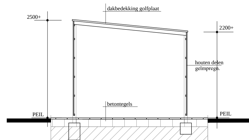
- ZIJGEVEL -
