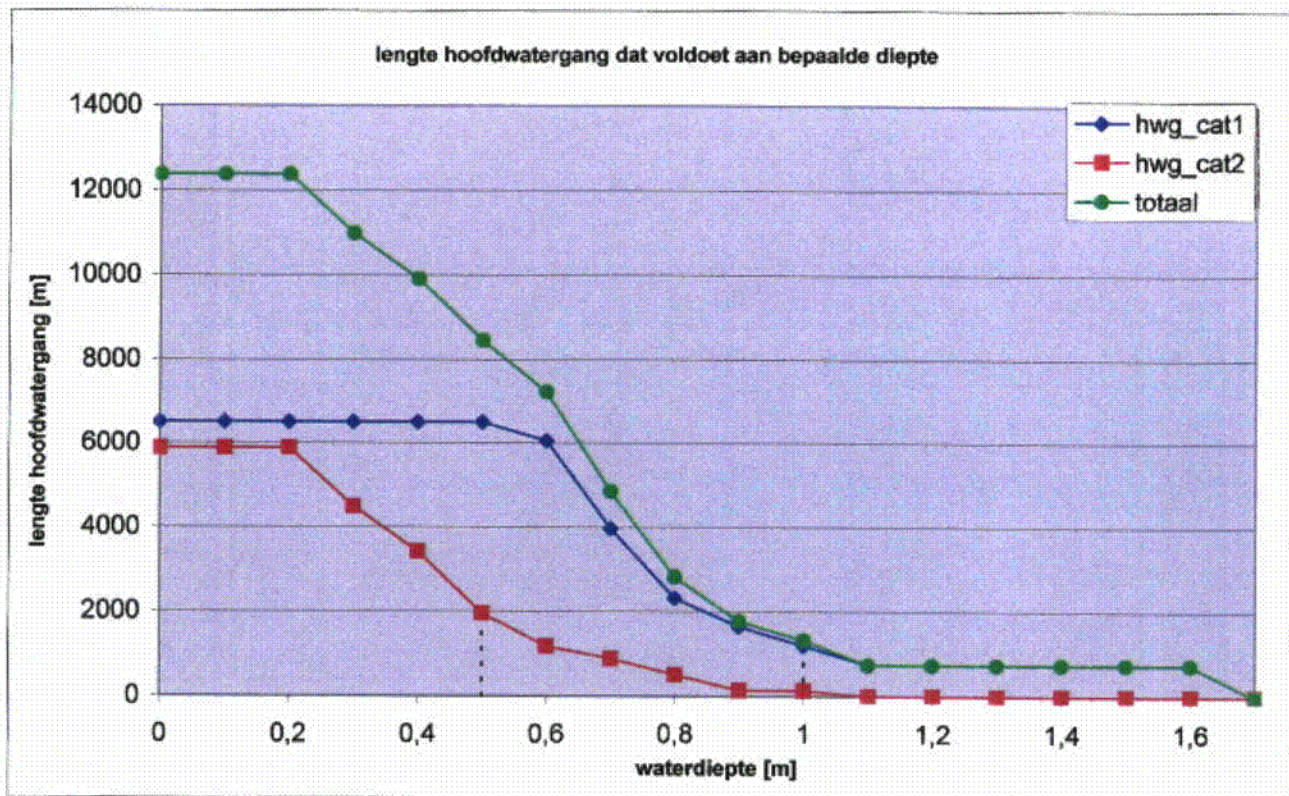
Bijlage 2a: Lengte en percentage hoofdwatrgang dat voldoet aan gegeven diepte
