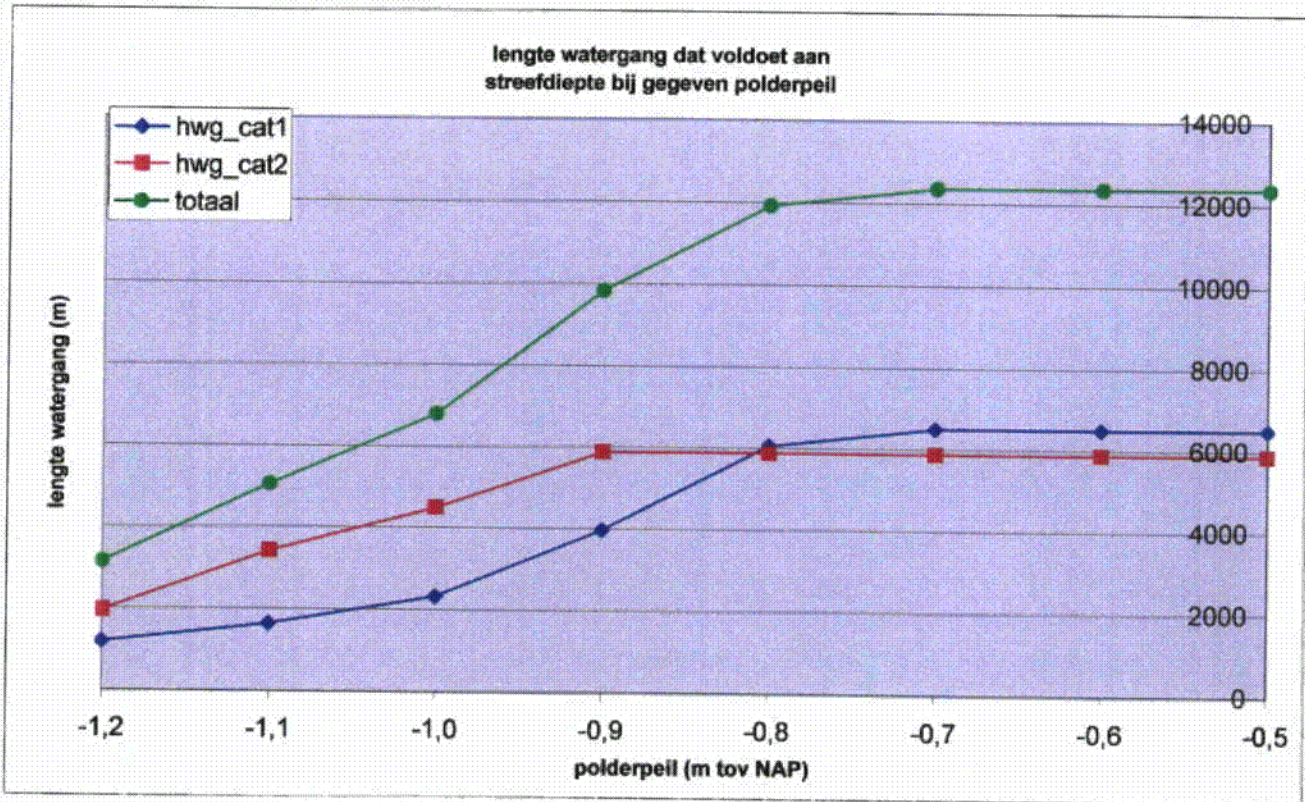
Bijlage 2b: Lengte en percentage hoofdwatrgang dat voldoet aan streefdiepte bij gegeven peilverhoging
