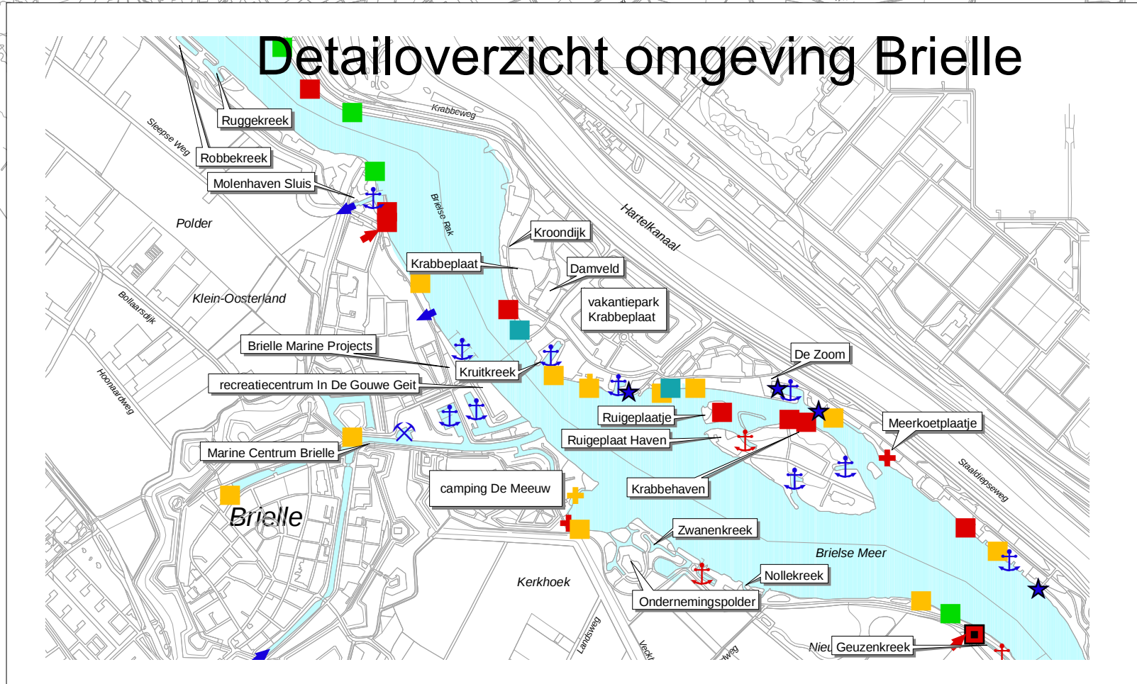
Overzicht peilschalen en meetpunten waterniveau
