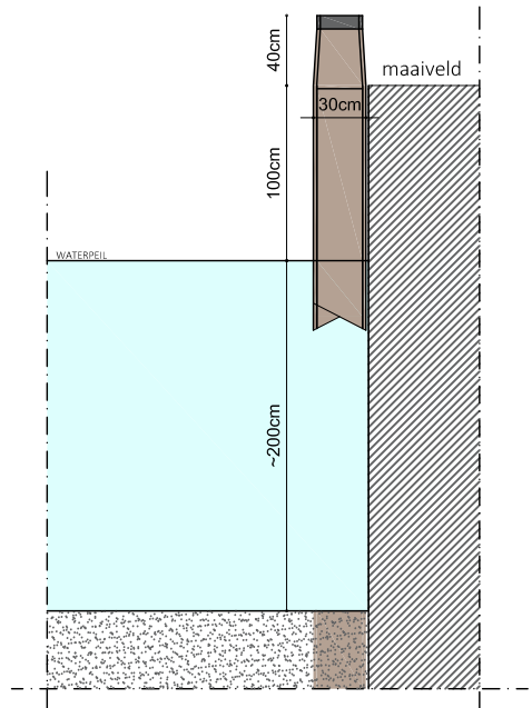
aanmeerpaal laag
