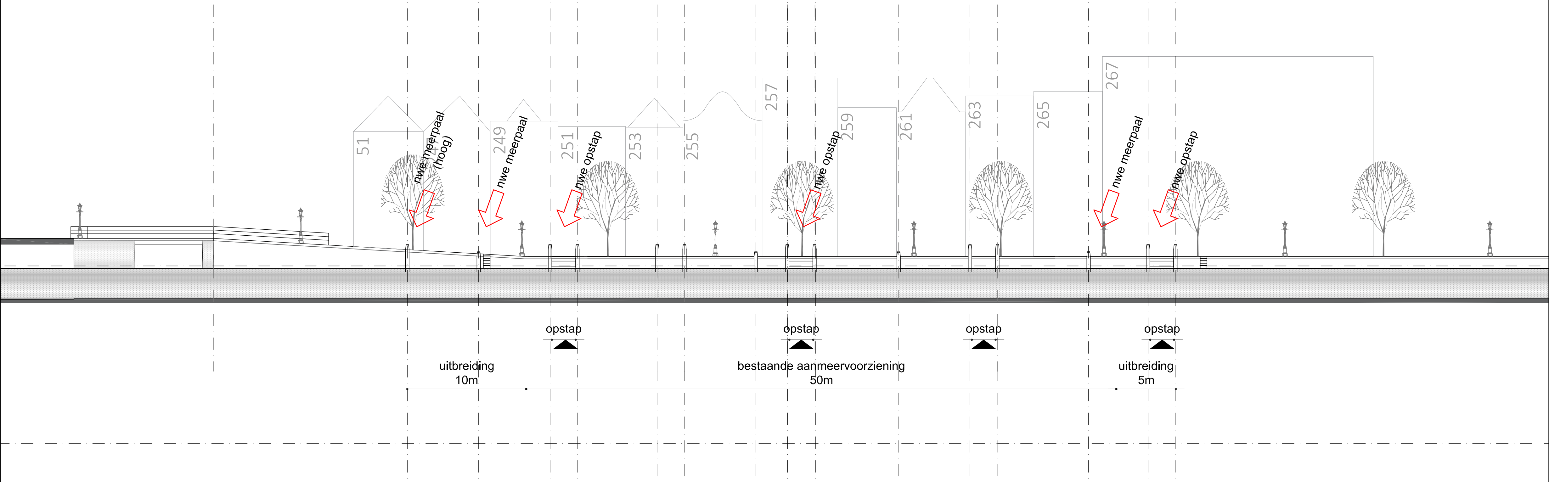
aanzicht kade schaal 1:200
