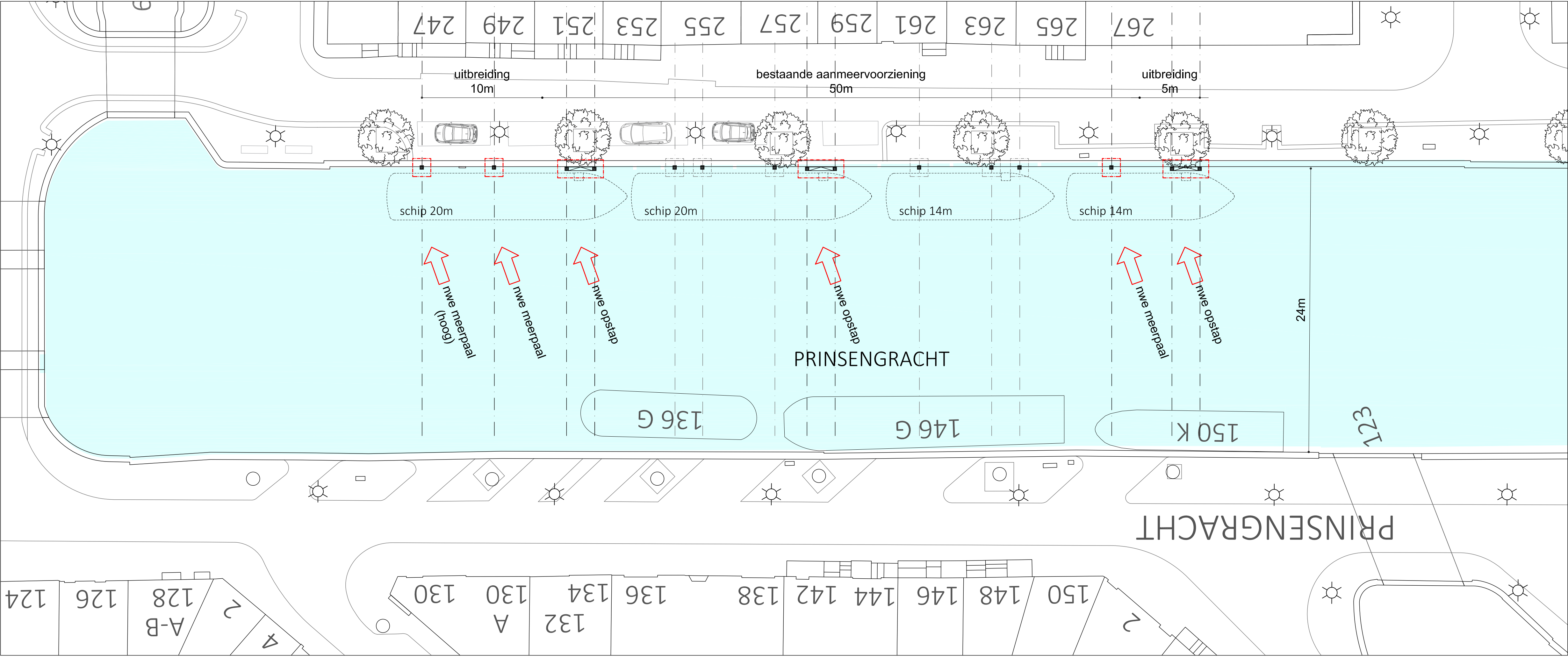
bovenaanzicht schaal 1:200
