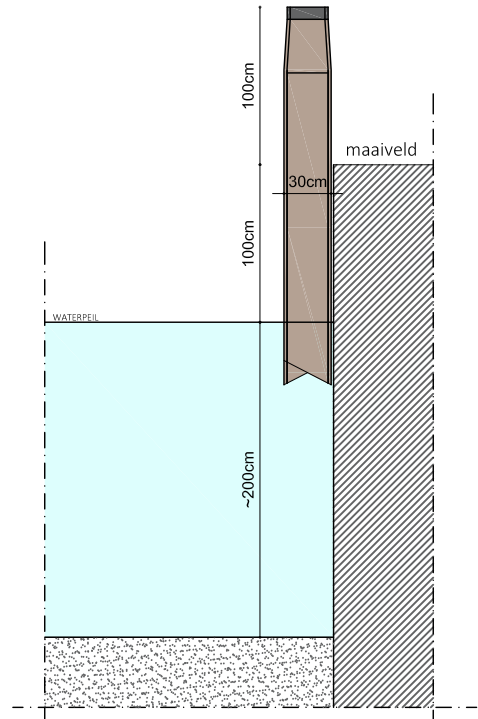
aanmeerpaal hoog
