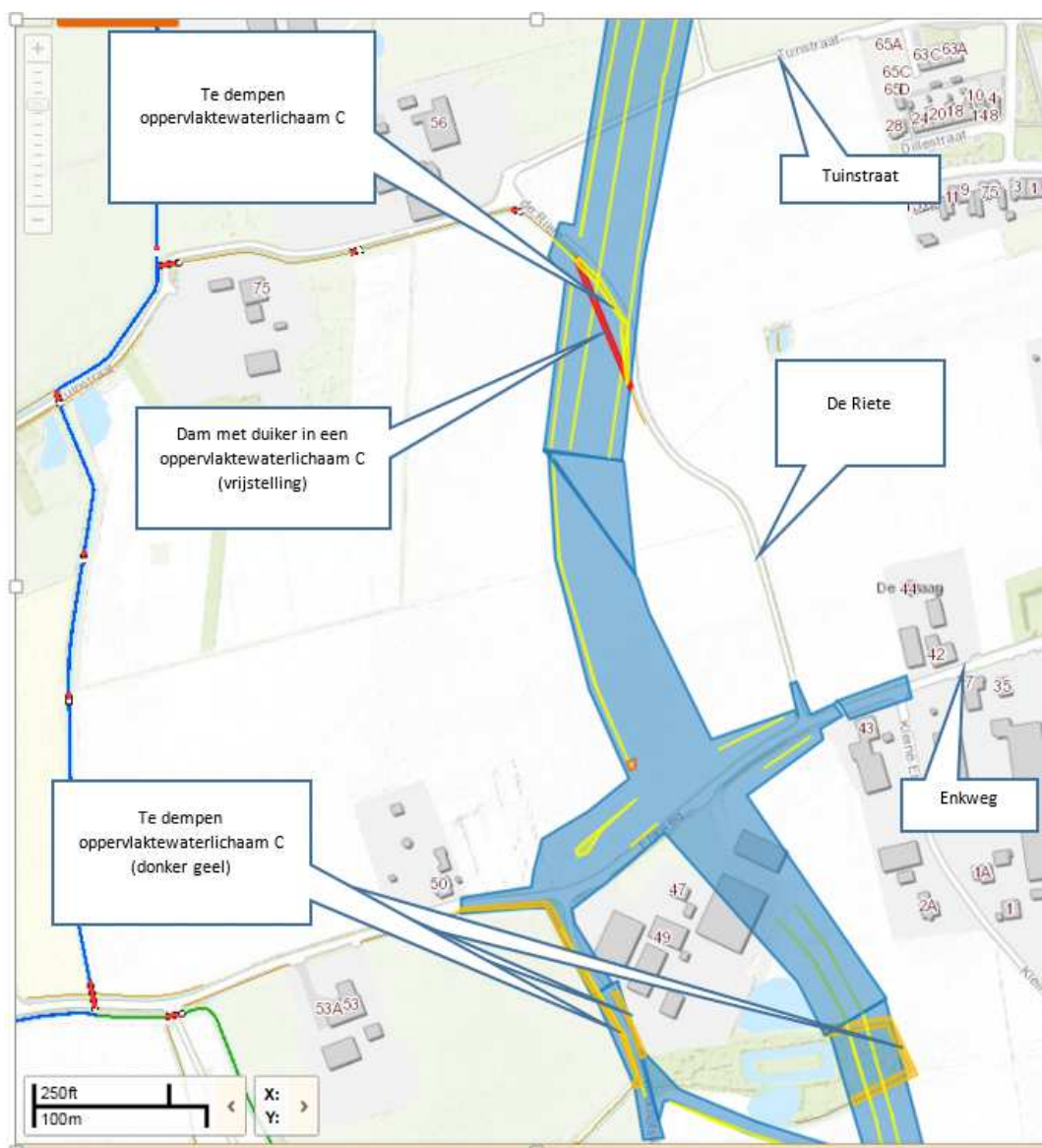
Tekening 4: Midden deel rondweg Voorst. De lichte gele lijnen zijn aan te leggen waterbergingen.
