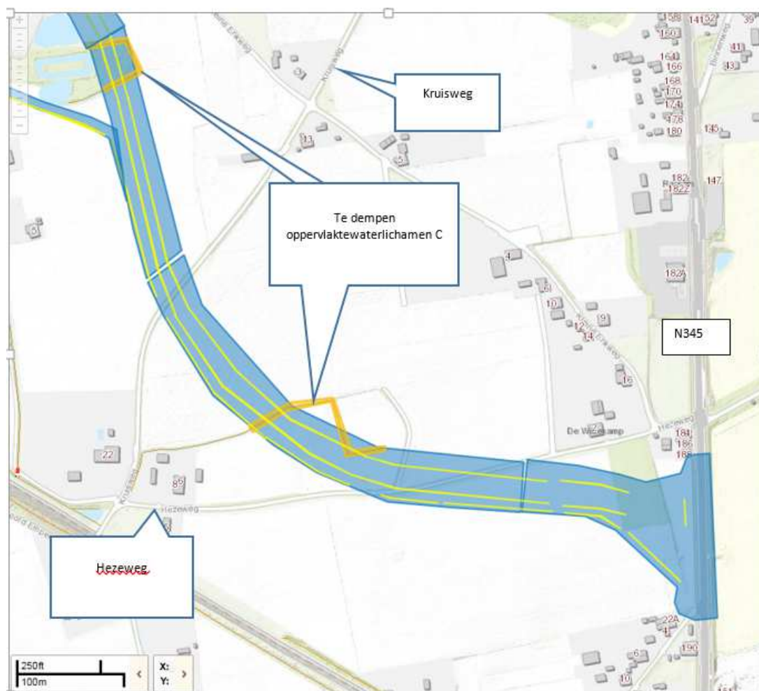
Tekening 4: Zuidelijk deel rondweg Voorst. De lichte gele lijnen zijn aan te leggen waterbergingen.
