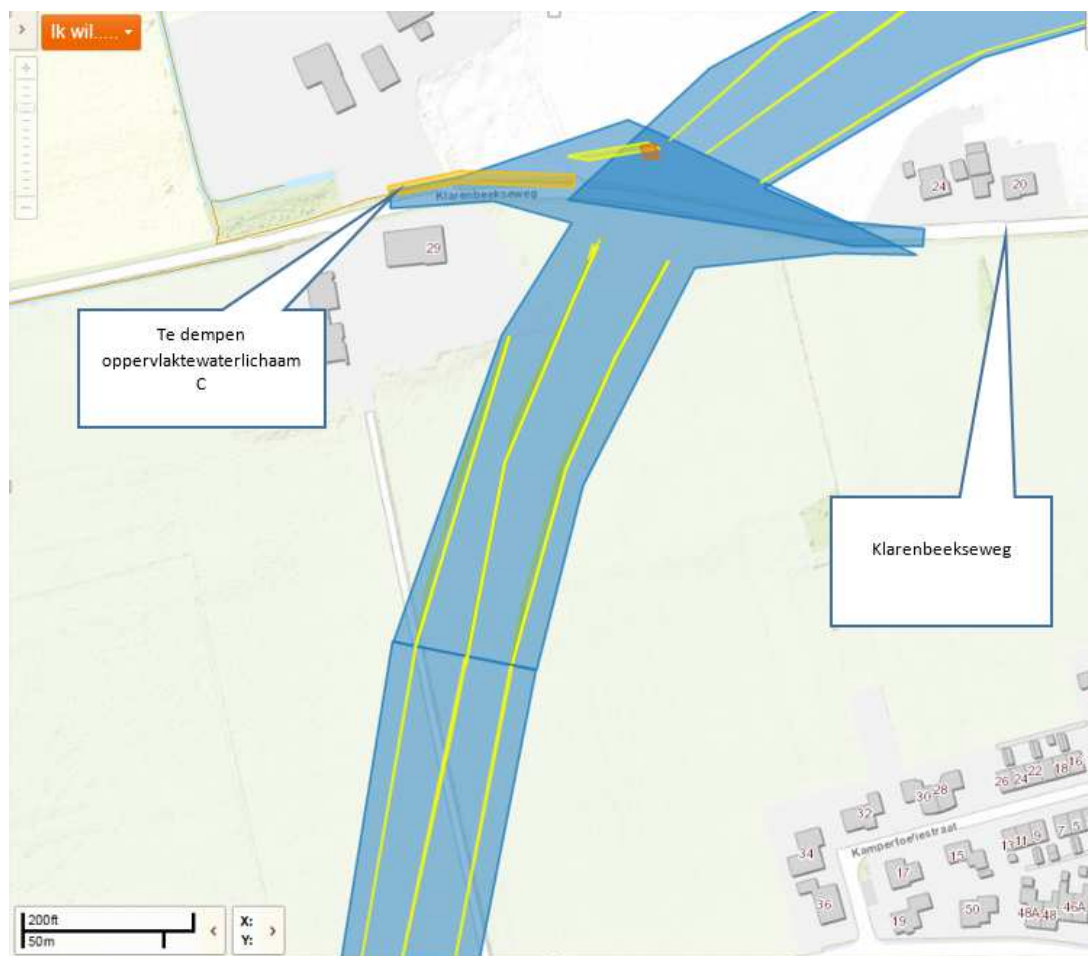
Tekening 3: Midden deel rondweg Voorst. De licht gele lijnen zijn aan te leggen waterbergingen.
