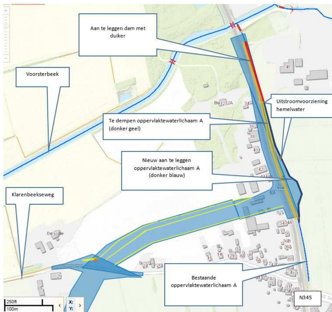
Tekening 2: Noordelijke deel rondweg Voorst. De lichte gele lijnen zijn aan te leggen waterbergingen.
