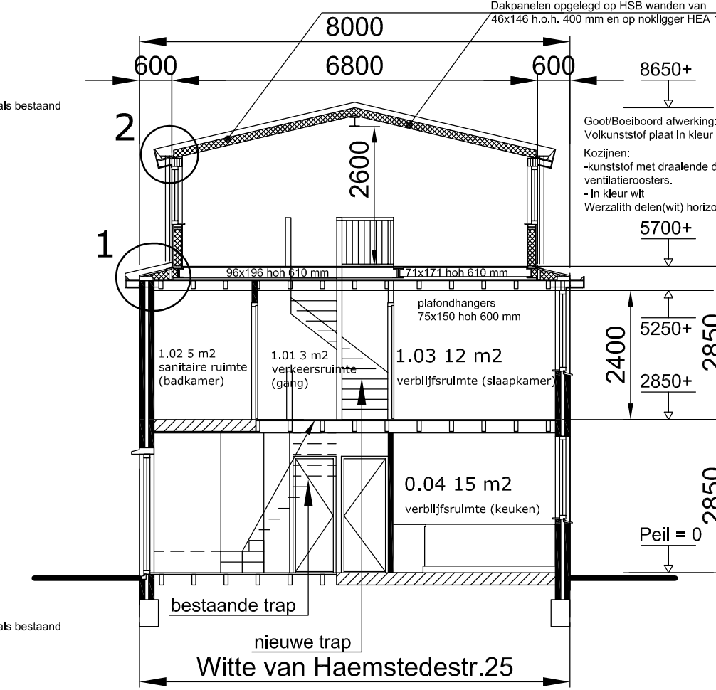
Doorsnede NIEUW
