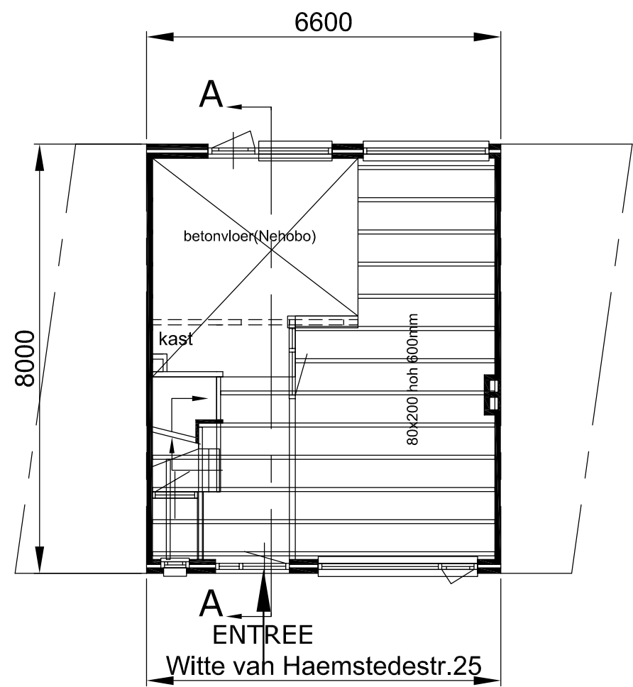
Begane grond BESTAAND balklaag
