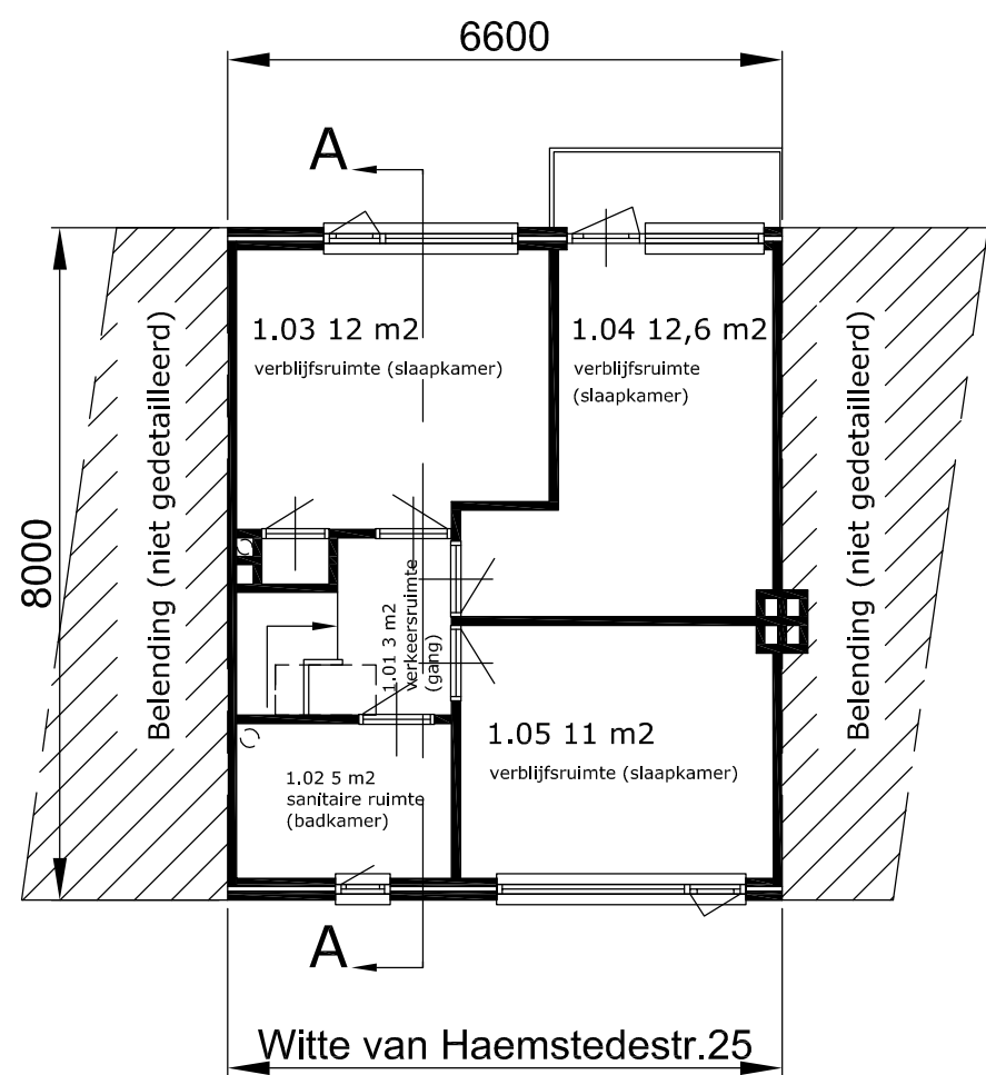
1e verdieping BESTAAND
