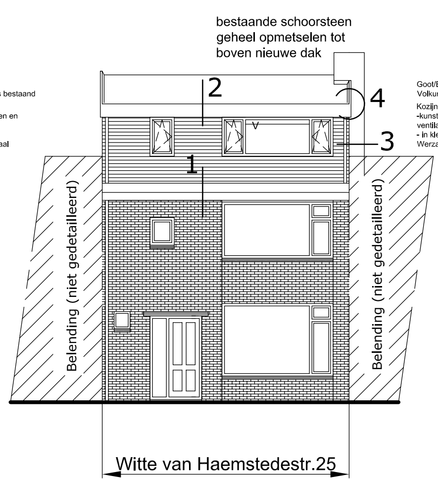
Voorgevel NIEUW
