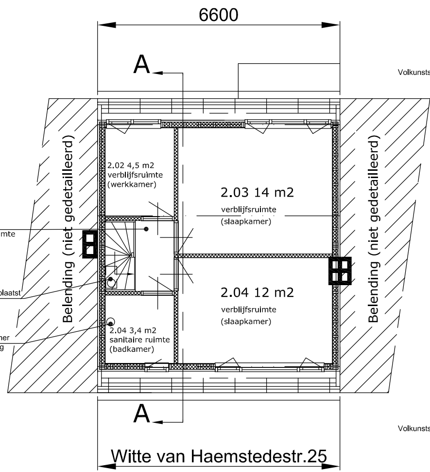
2e Verdieping NIEUW
