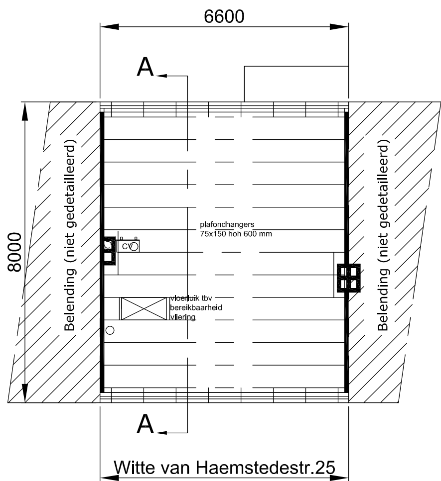
Vliering BESTAAND
