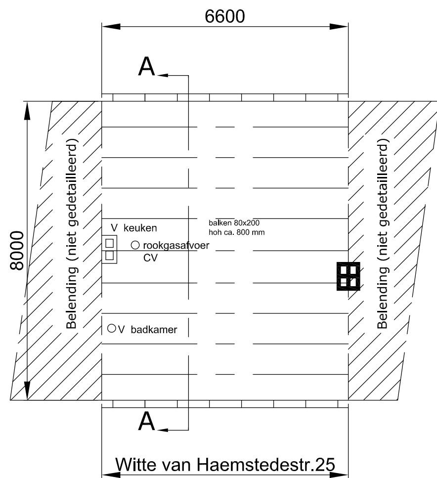
Dak BESTAAND
