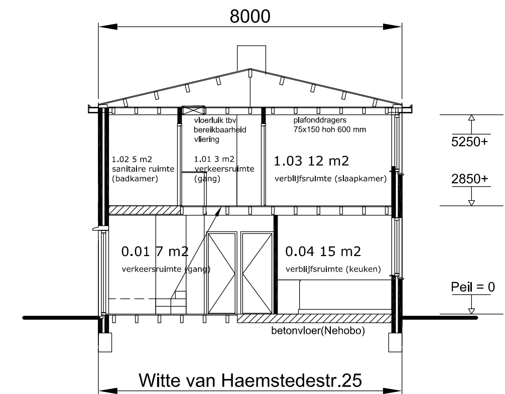
Doorsnede BESTAAND
