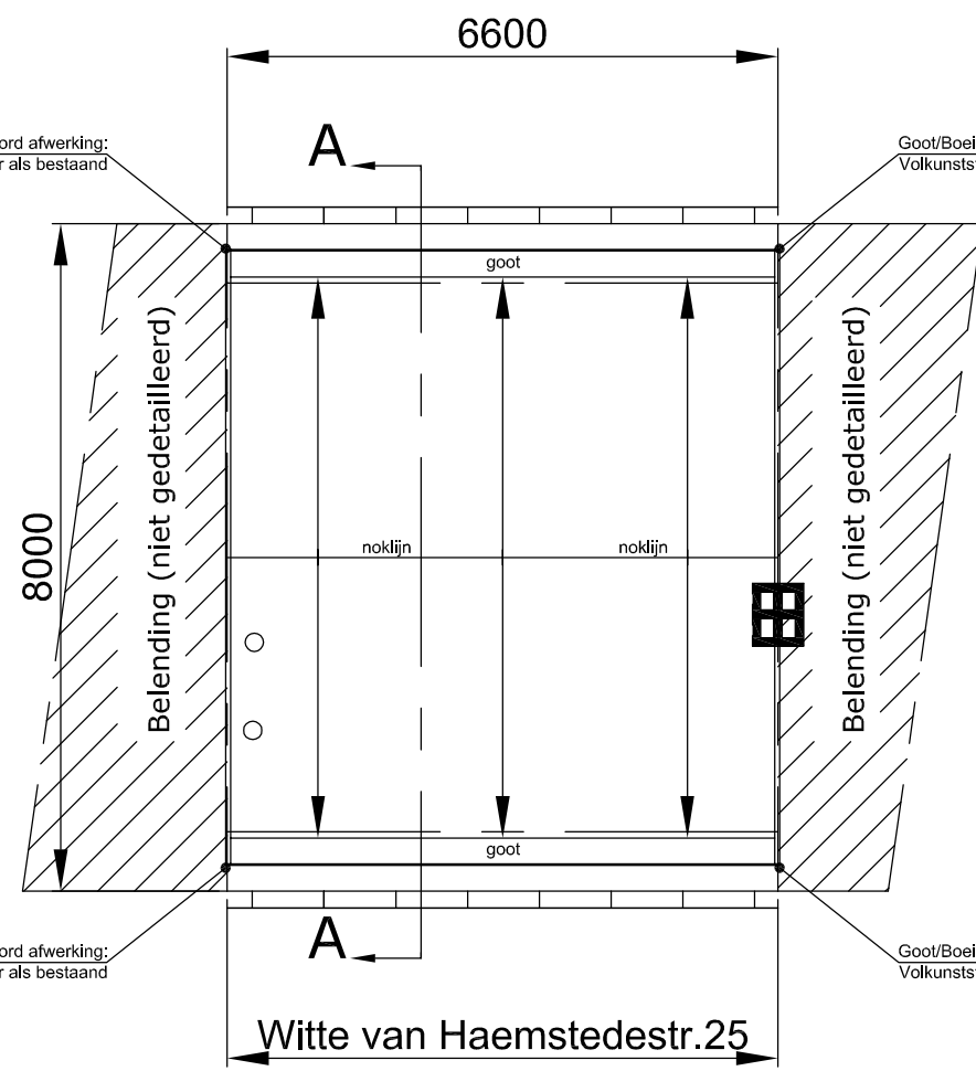
Dak NIEUW
