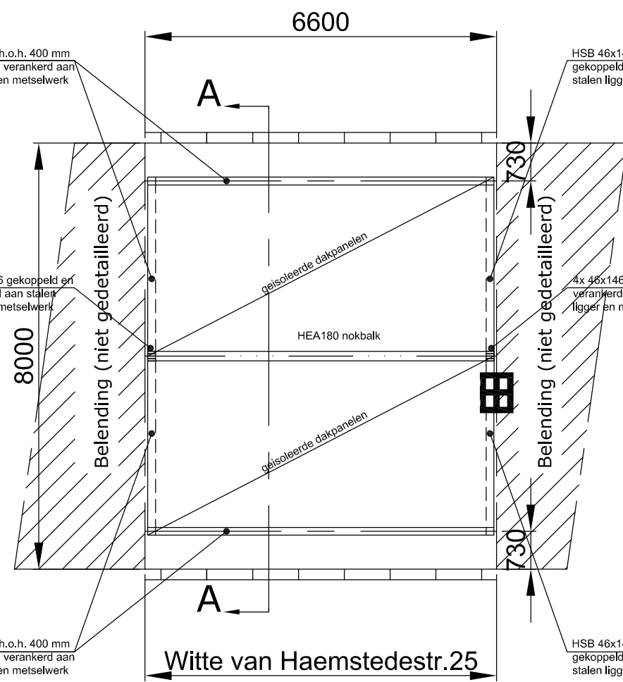
Dak NIEUW constructieve ligger en dakpanelen
