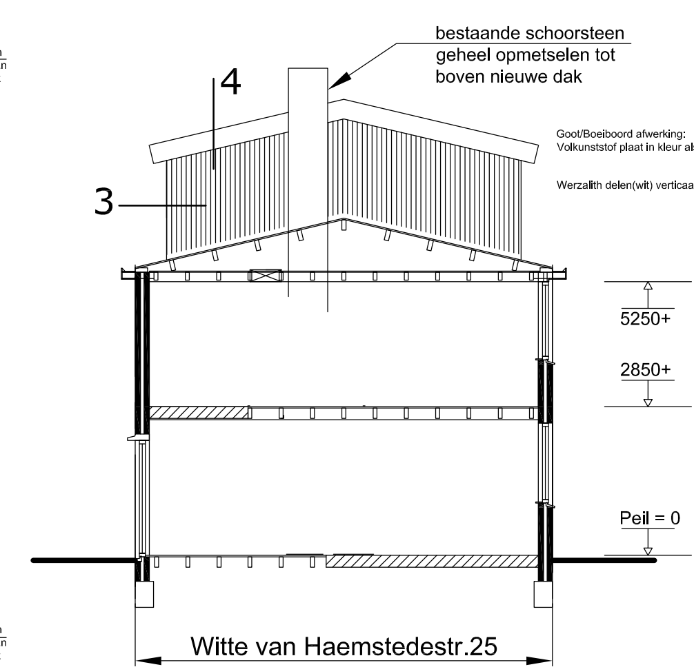
Doorsnede BELENDING Aanzicht kopgevel
