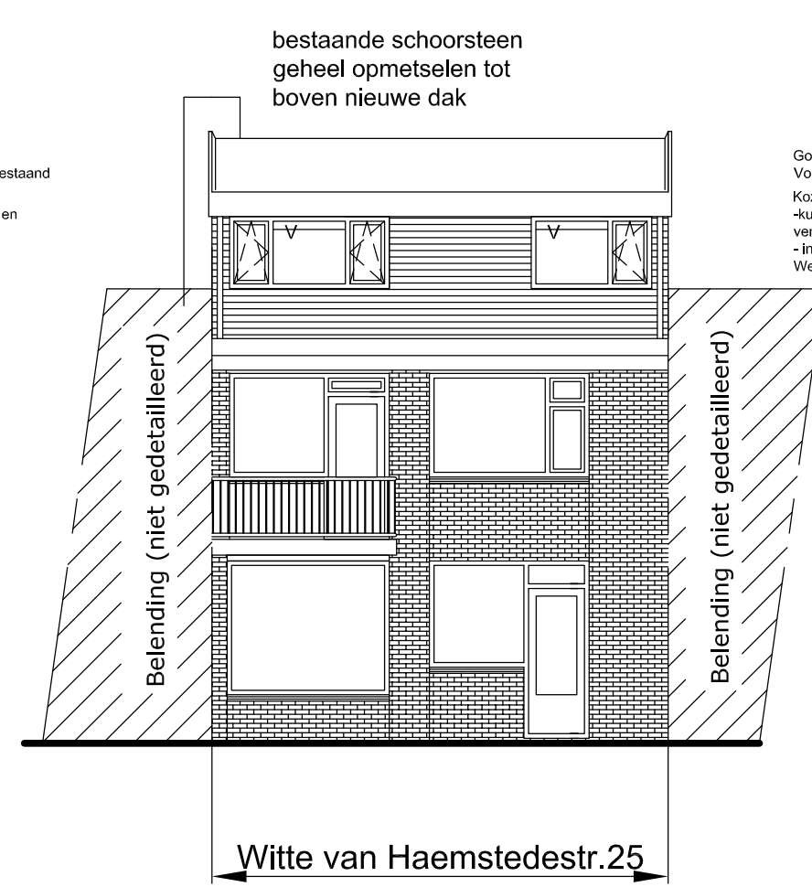
Achtergevel NIEUW
