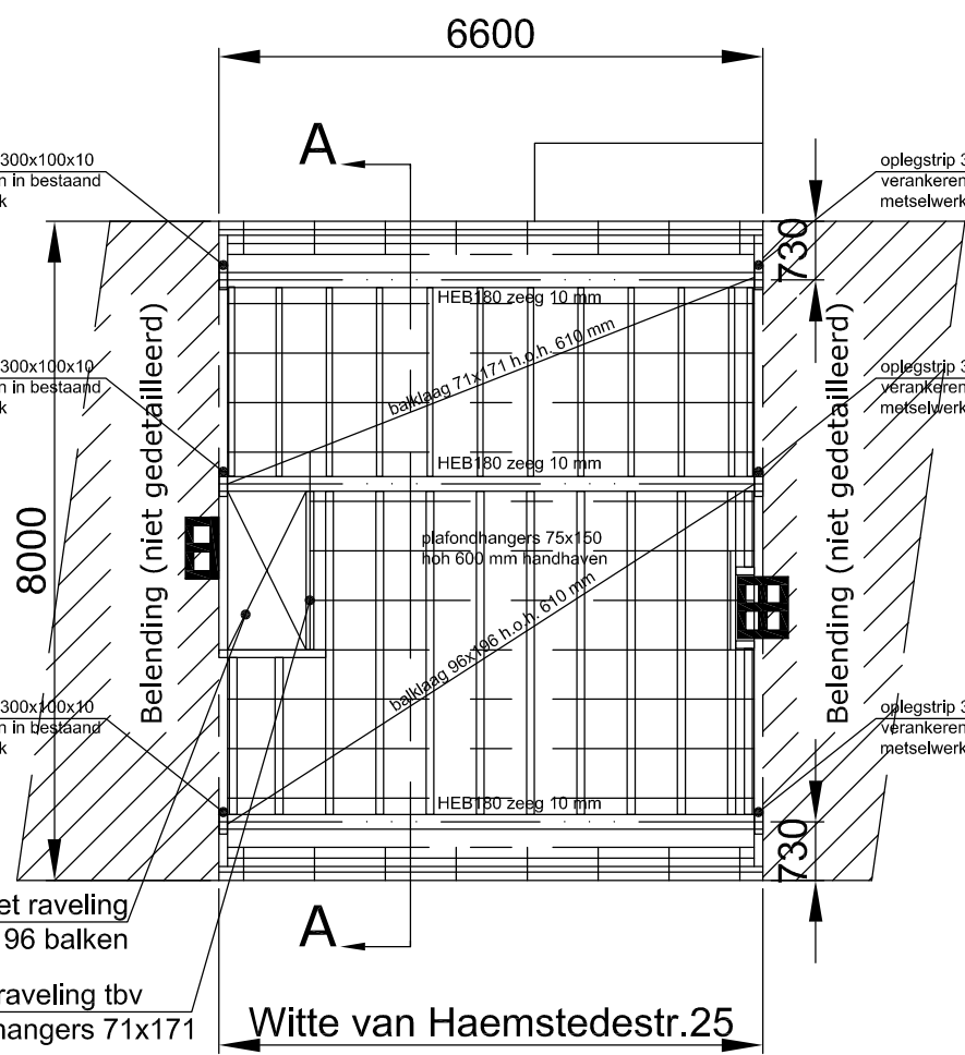
2e Verdieping NIEUW constructieve liggers en houten balklaag
