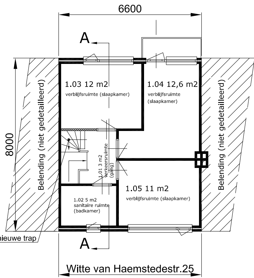
1e verdieping NIEUW
