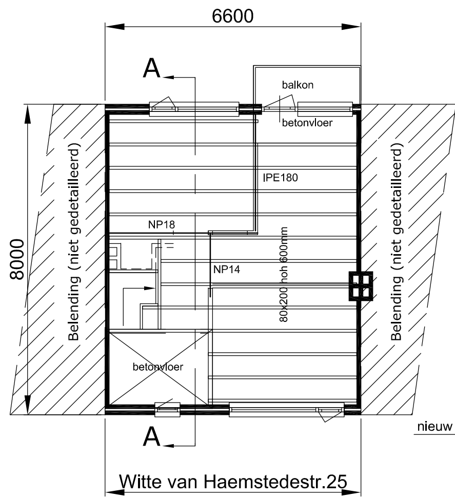
1e verdieping BESTAAND balklaag
