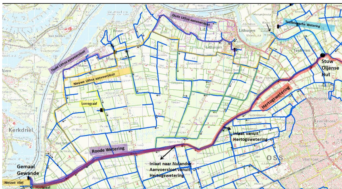
Figuur 2.1 Schets van het watersysteem van de Hertogswetering en de Roode Wetering
