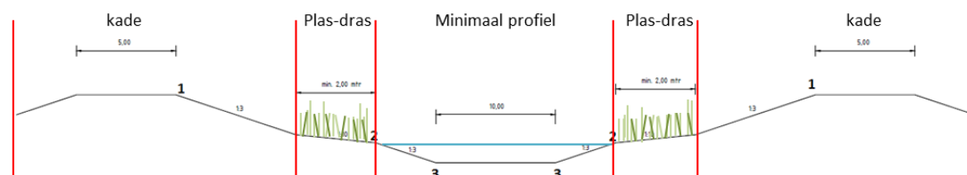
Figuur 2.2 Minimum profiel van de Hertogswetering
