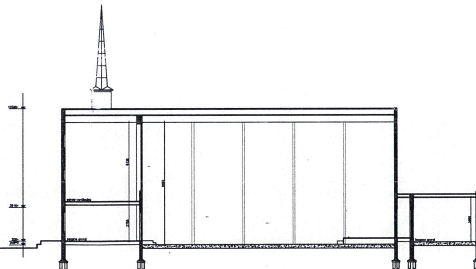
Doorsnede C-C
