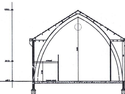
Doorsnede A-A
