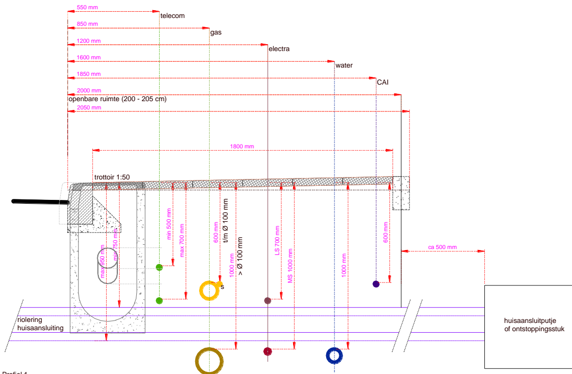
Profiel 1, breedte 200 cm (bestaande trottoirs in bestaande wijken) Kenmerk: breed trottoir
