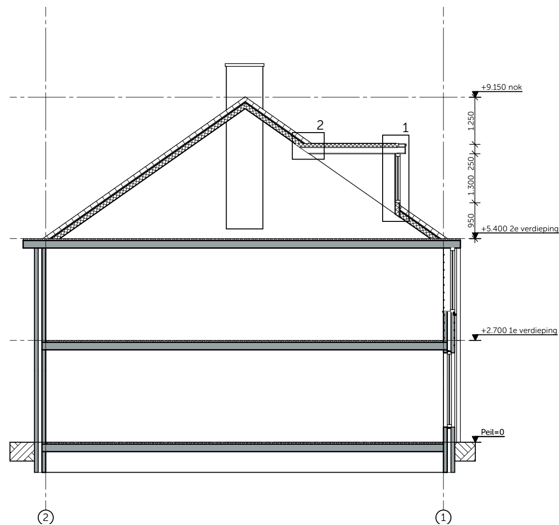
doorsnede A nieuw
