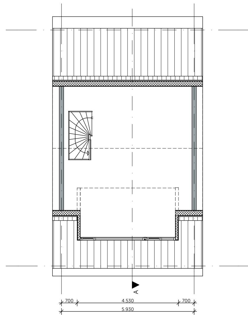
2e verdieping nieuw
