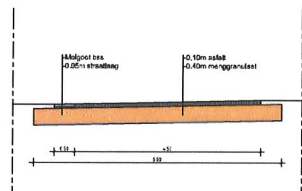
Principe doorsnede weg schaal 1:50
