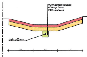
Principe doorsnede wadi schaal 1:50
