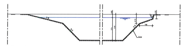
Principe doorsnede vijver schaal 1:50
