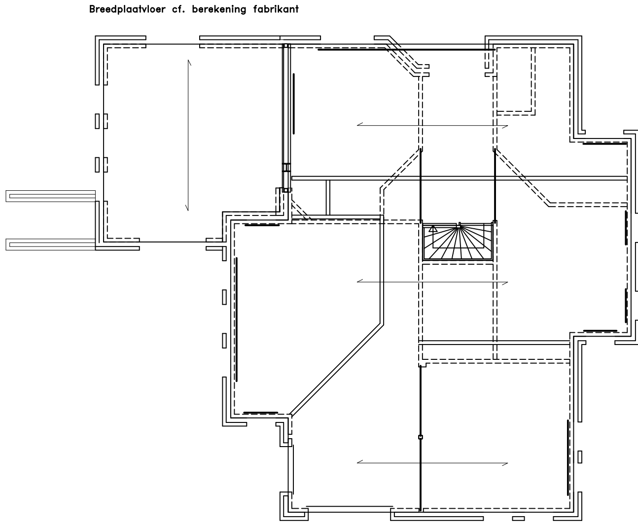
Verdiepingsvloer
