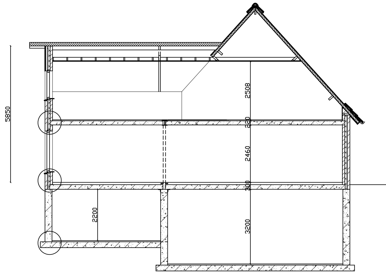
Doorsnede
