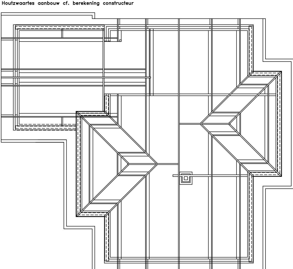
Kapconstructie
