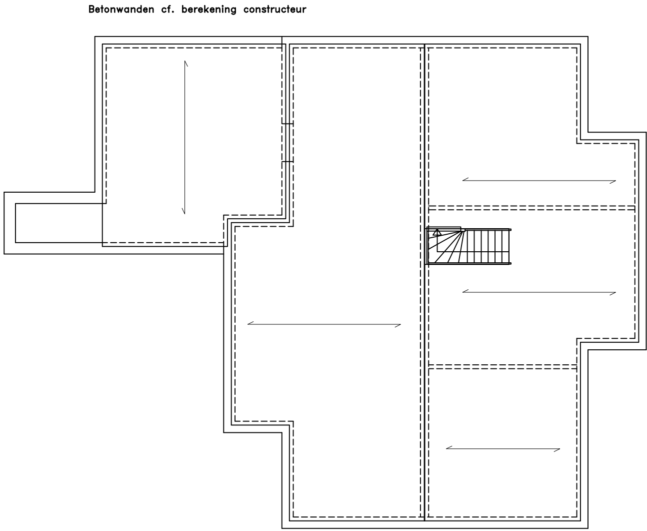
Begane grondvloer
