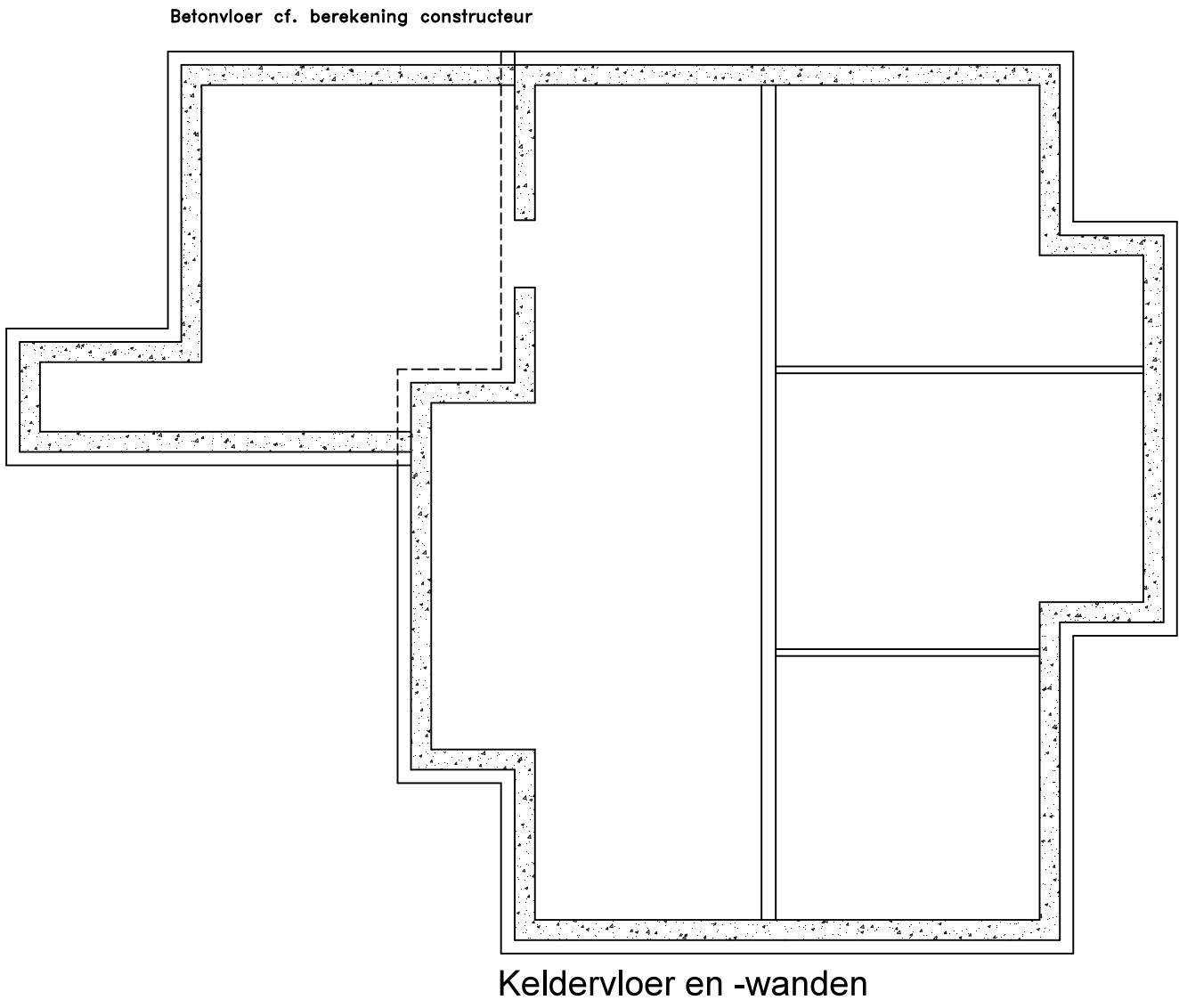
Keldervloer en -wanden
