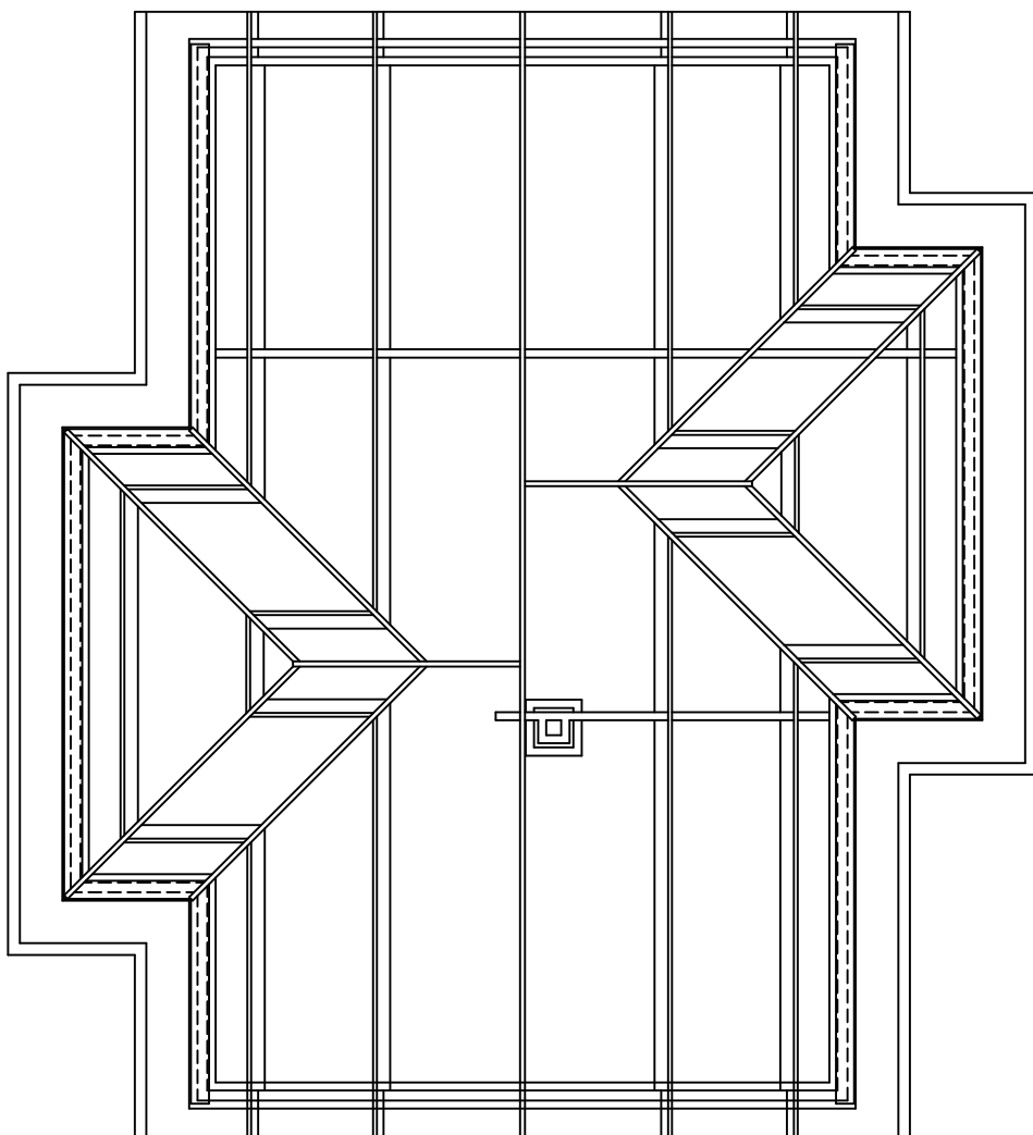
Kapconstructie
