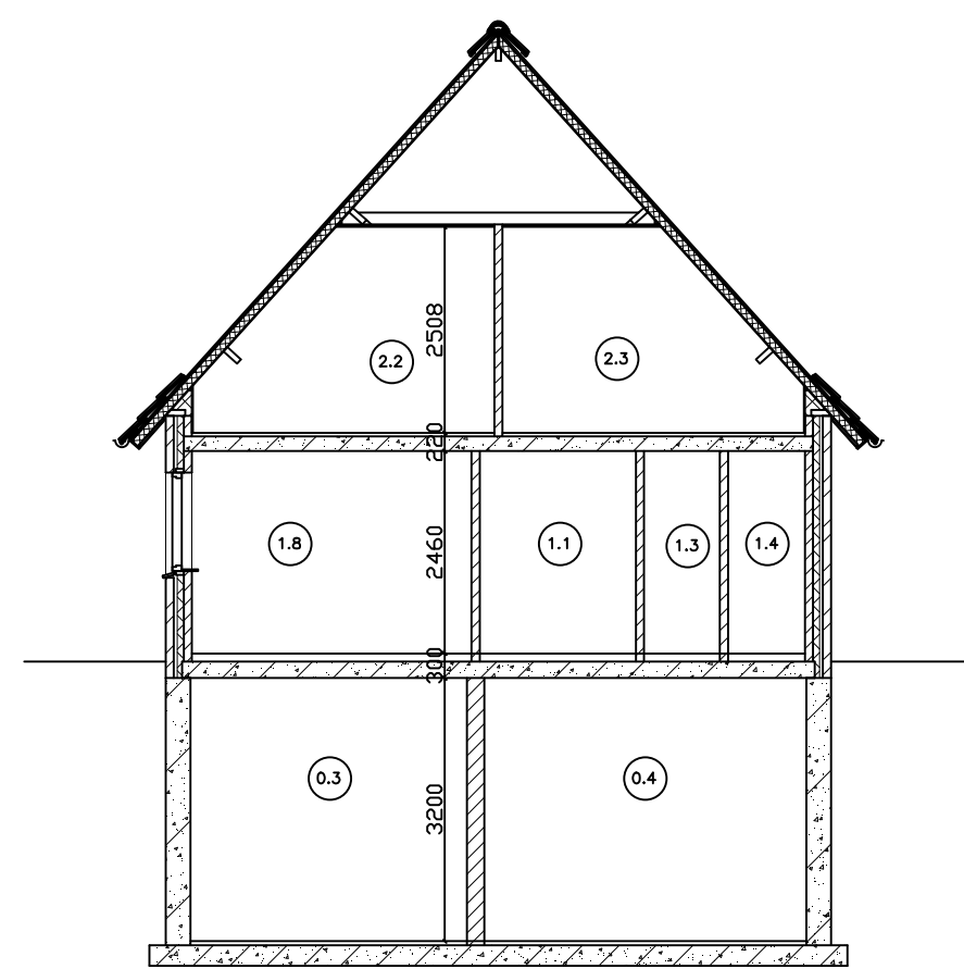
Doorsnede
