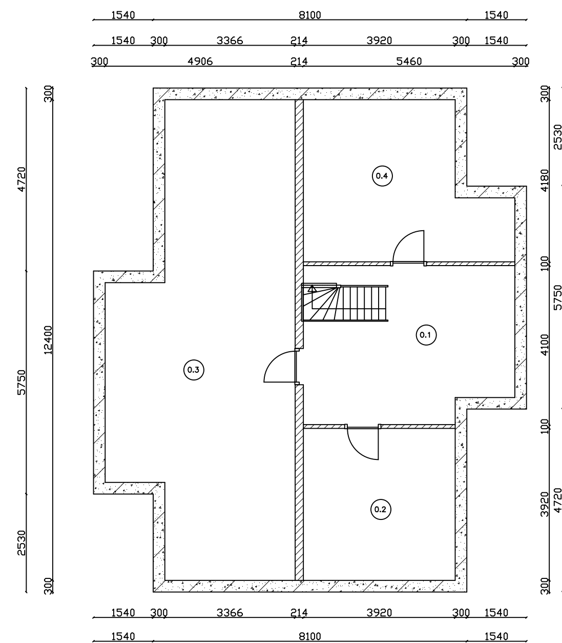
Kelder
