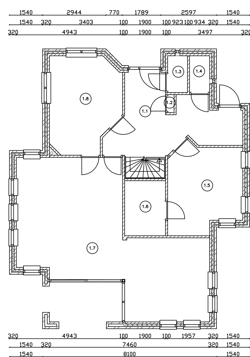
Begane grond
