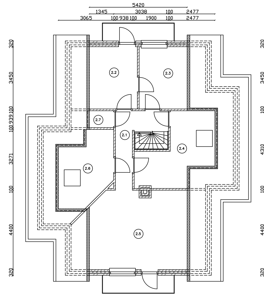
Verdieping
