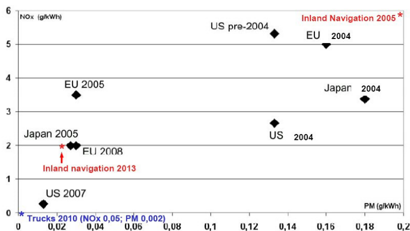
Figuur 3.2 Internationale emissienormen voor PM en NO x voor zware vrachtwagens en binnenvaart.
