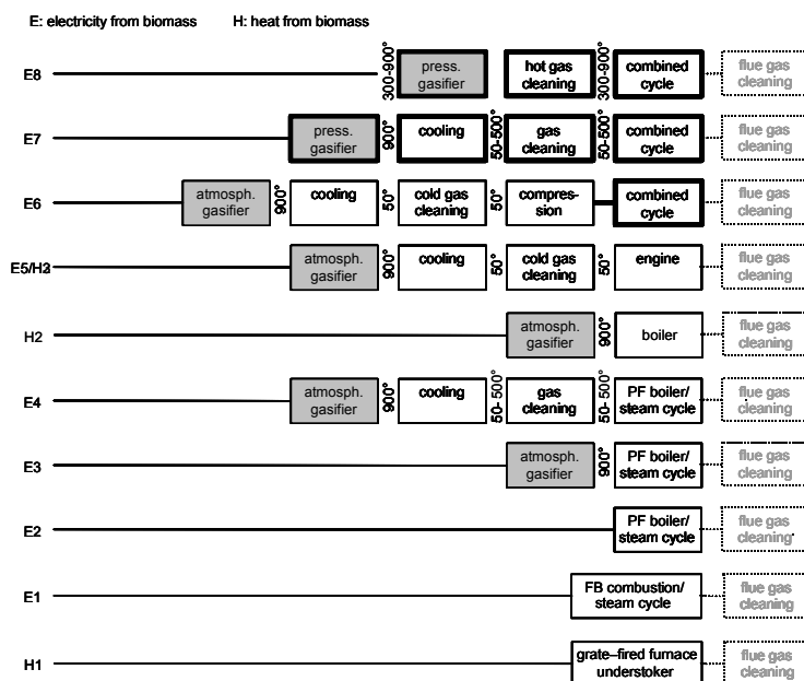
Figuur 4.1 Overzicht van de technologieën voor elektriciteit- en warmteopwekking uit biomassa
