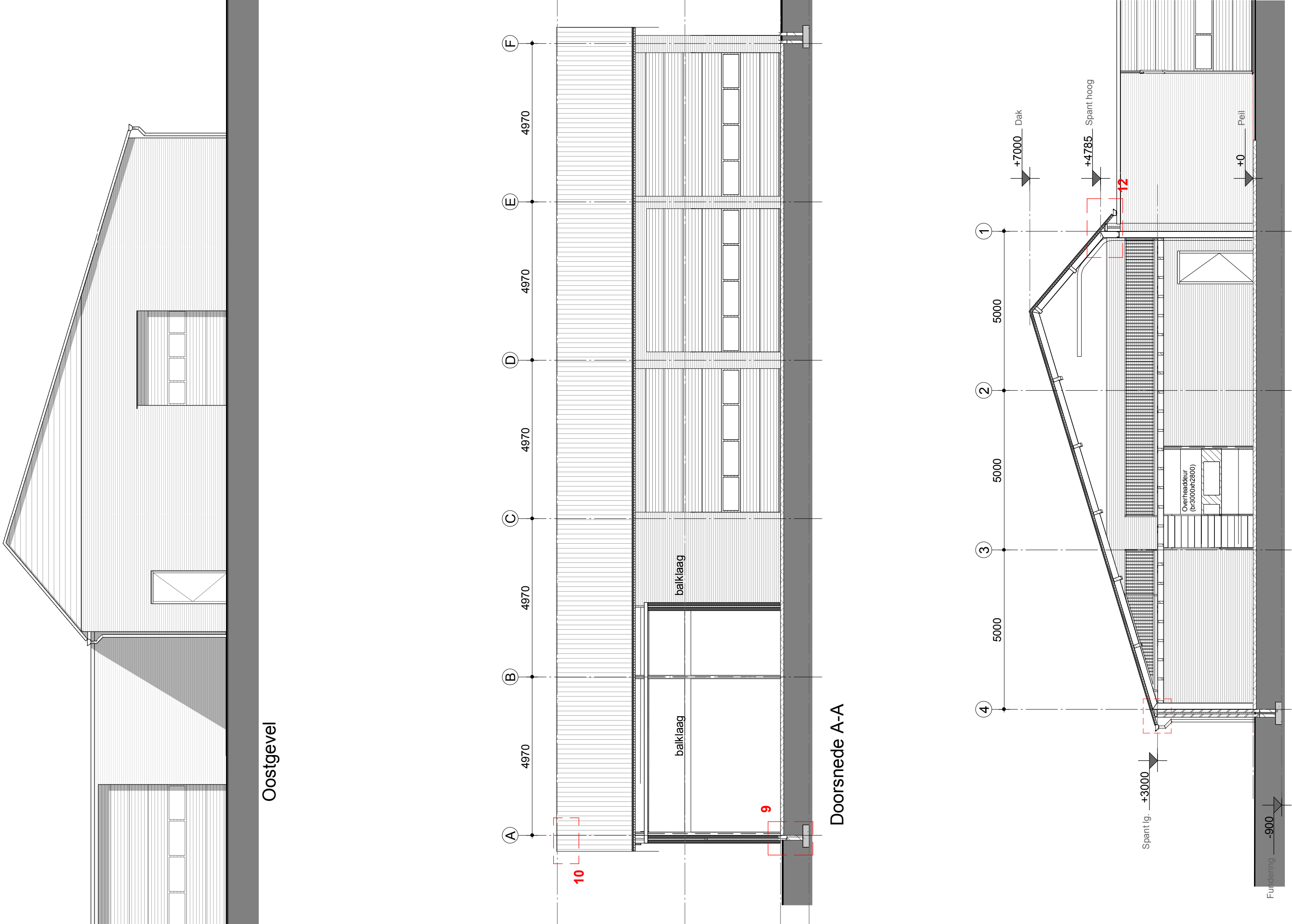
Doorsnede B-B
