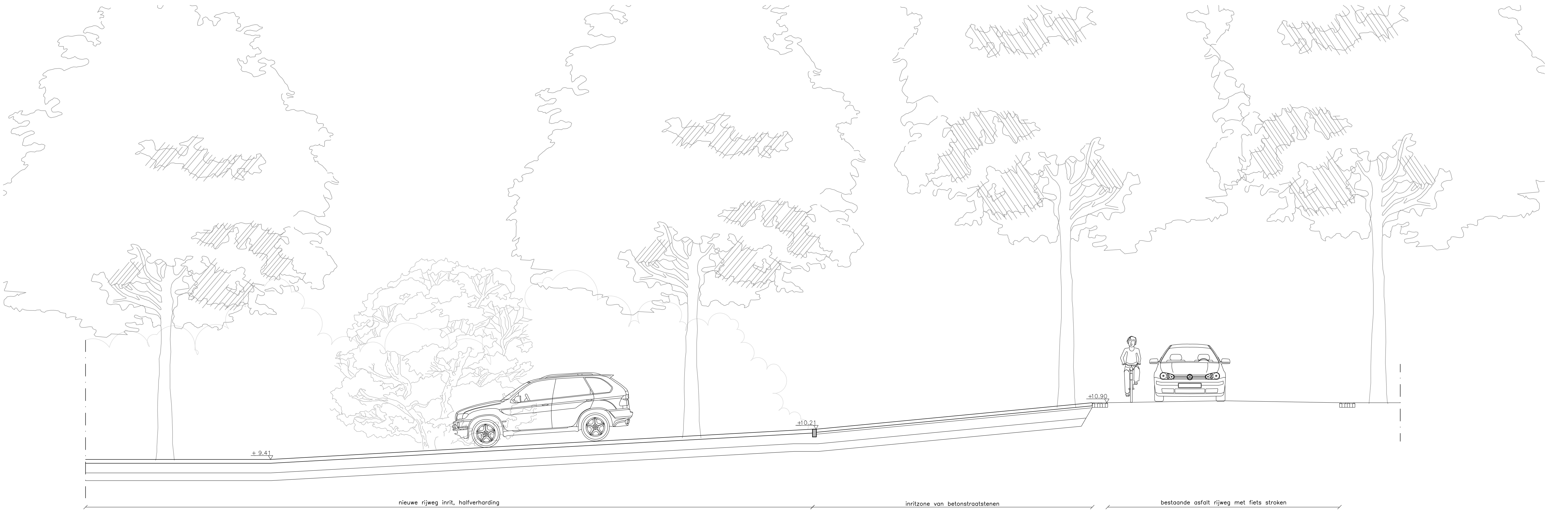
Langsdoorsnede nieuwe toerit schaal 1:50
