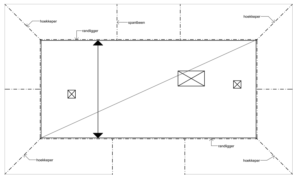
2E VERDIEPINGVLOER
