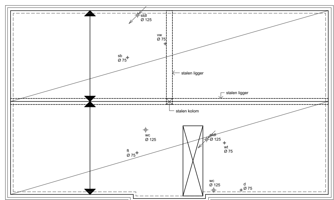
BEGANE GRONDVLOER
