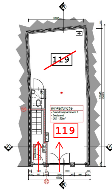
BEGANE GROND NIEUWE SITUATIE
