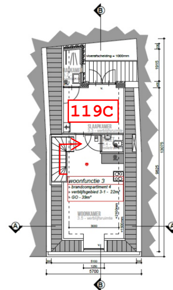
DERDE VERDIEPING NIEUWE SITUATIE
