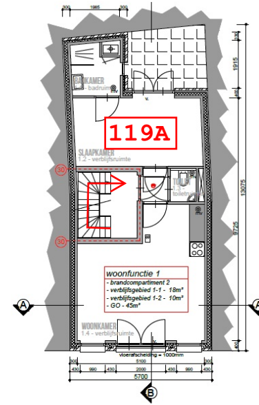
EERSTE VERDIEPING NIEUWE SITUATIE
