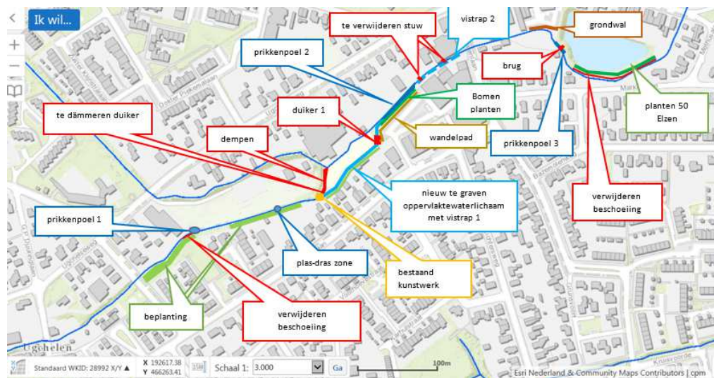
Situatietekening 1
