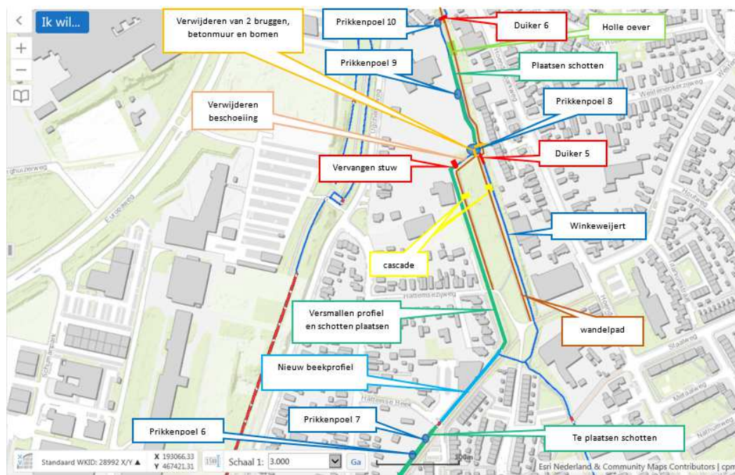
Situatietekening 3
