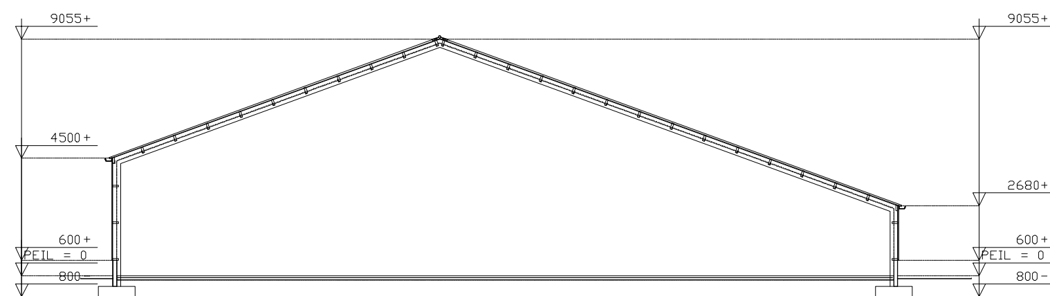
DOORSNEDE STAL 3
