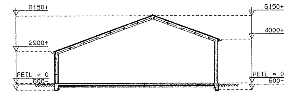
DOORSNEDE STAL 2
