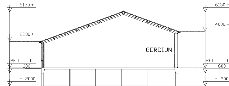
DOORSNEDE STAL 2
