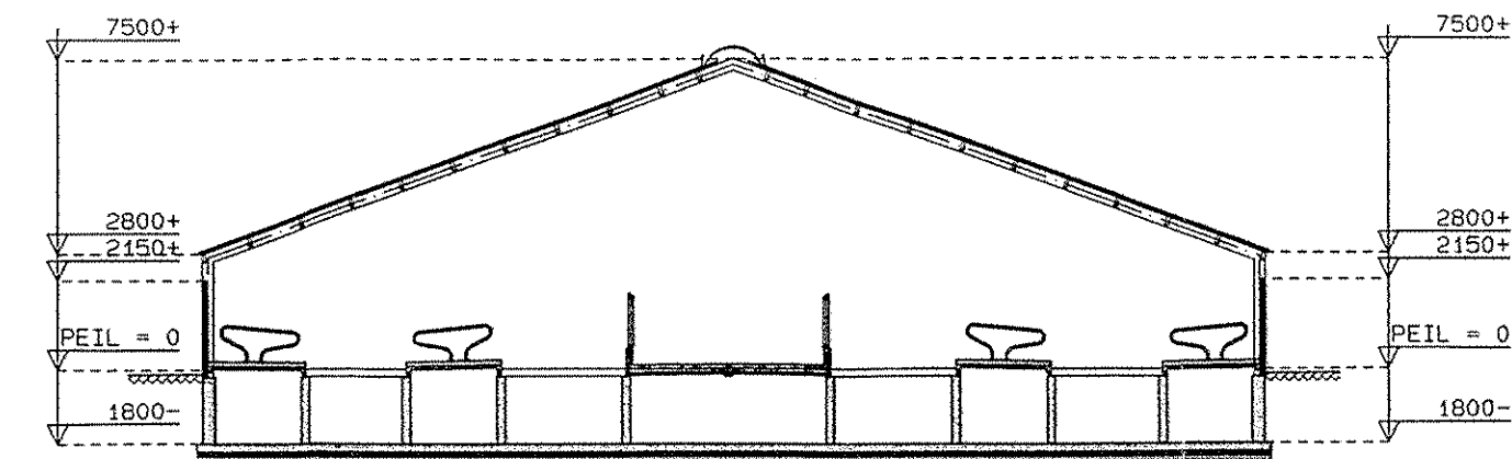
DOORSNEDE STAL 1
