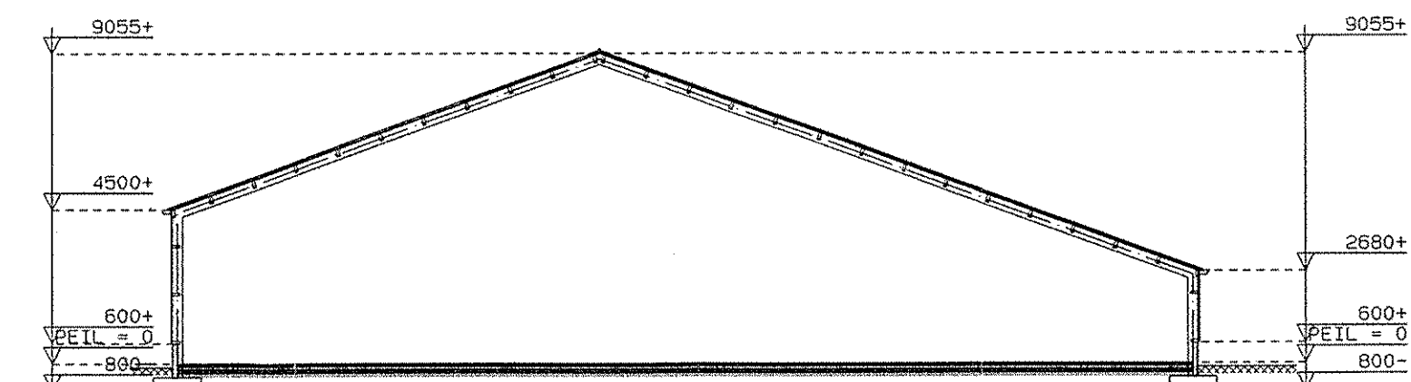
DOORSNEDE STAL 3
