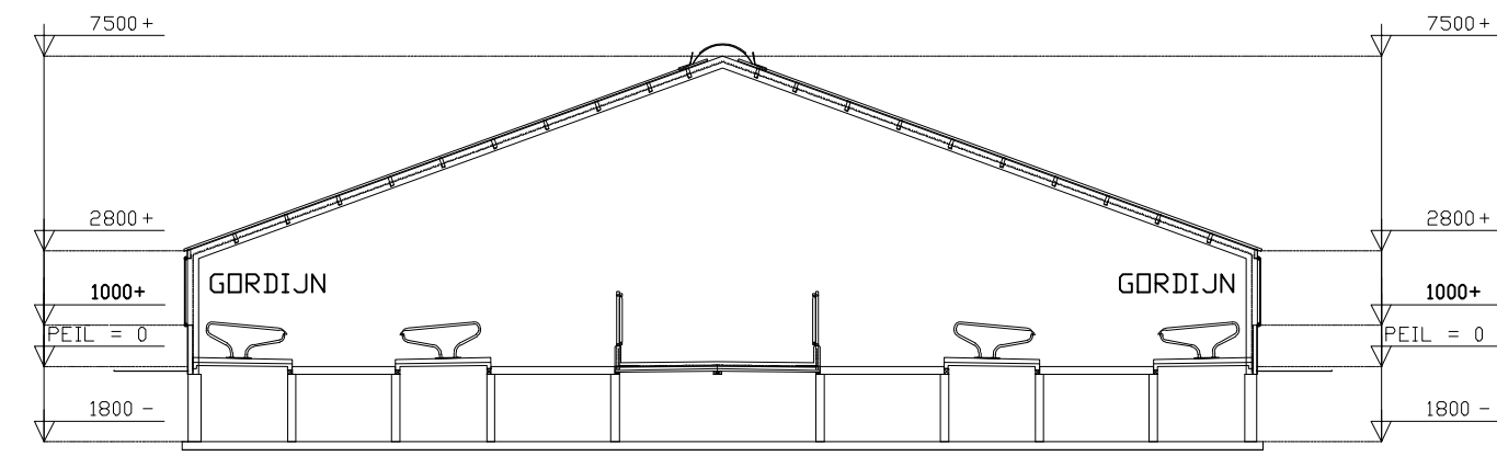
DOORSNEDE STAL 1
