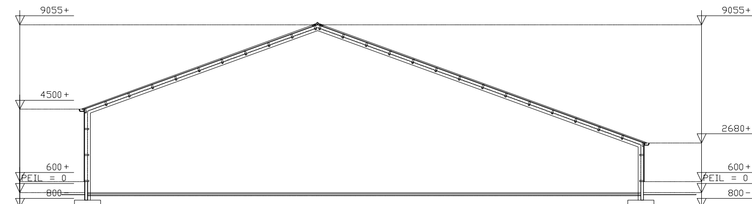
DOORSNEDE STAL 3
