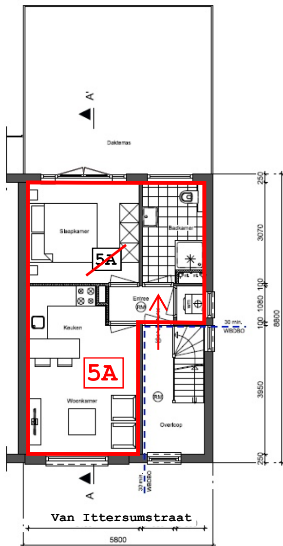
Verdieping (nieuw)
