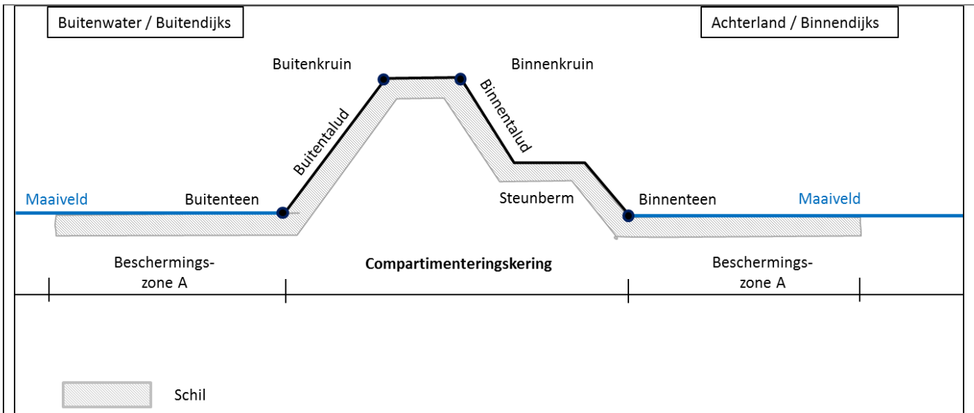
Figuur 25A.1: ligging schil compartimenteringskering
