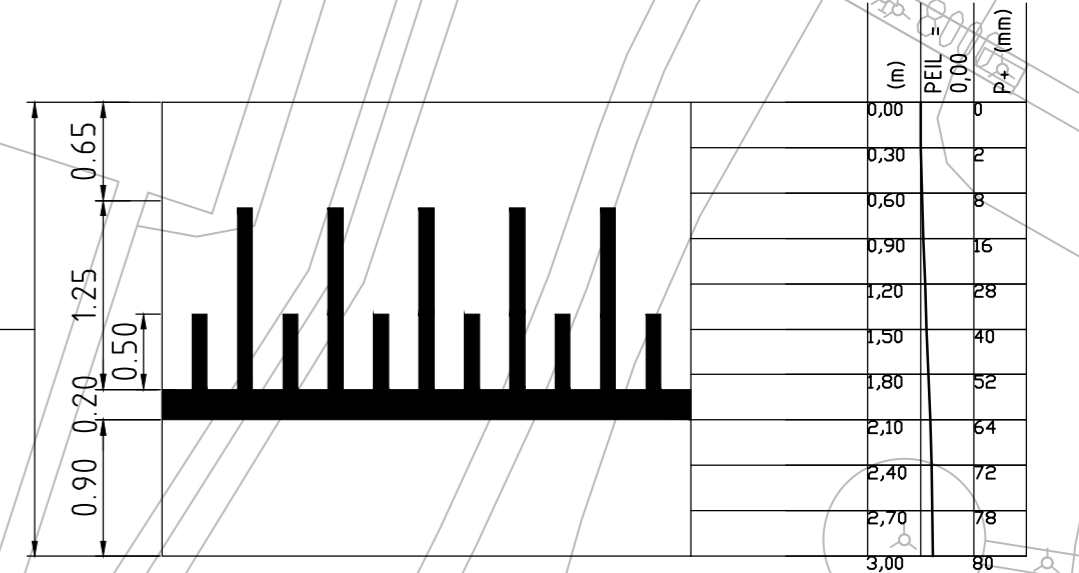
PRINCIPEDETAIL DREMPELCONSTRUCTIE 50KM/UR, HOOGTE 8CM, ROOD ASFALT
