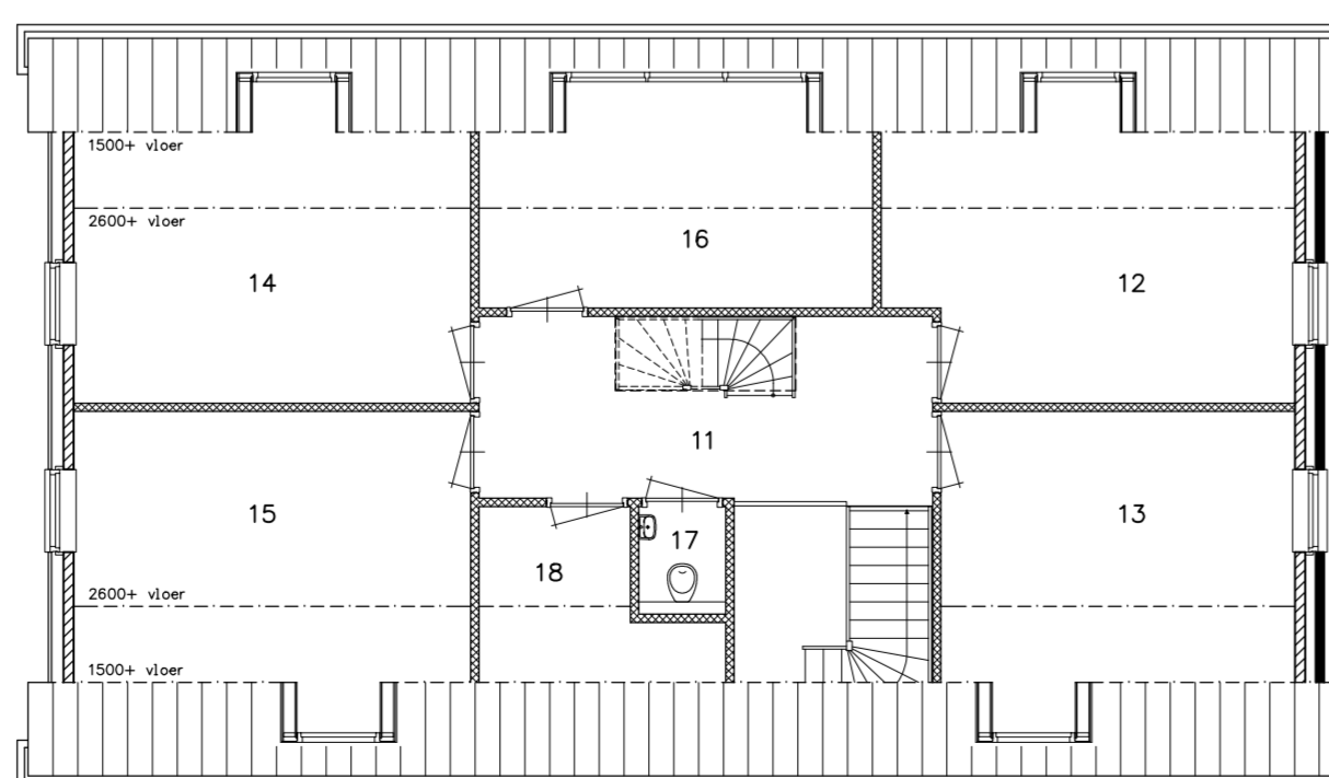
Verdieping
