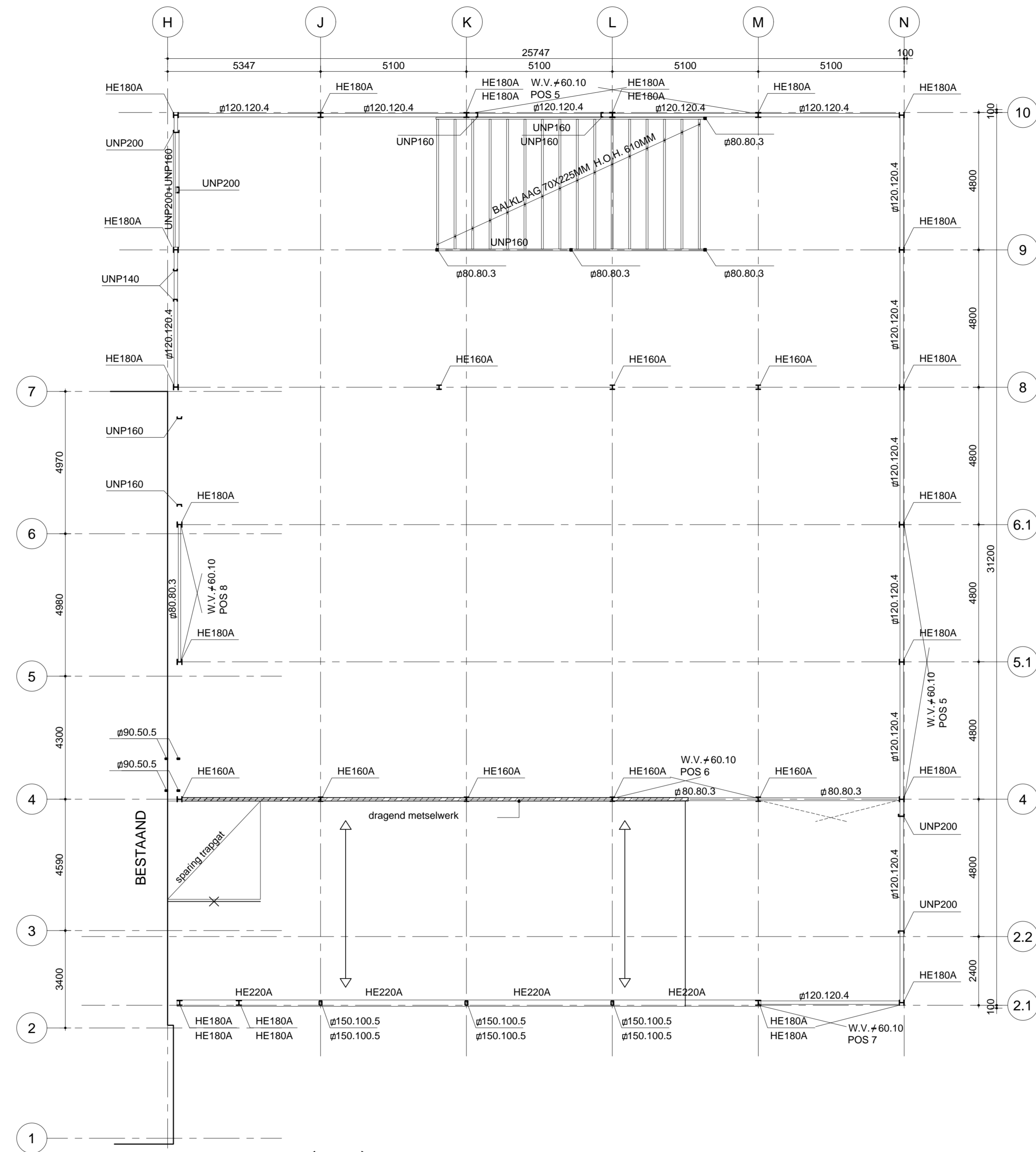
VERDIEPINGSVLOER
