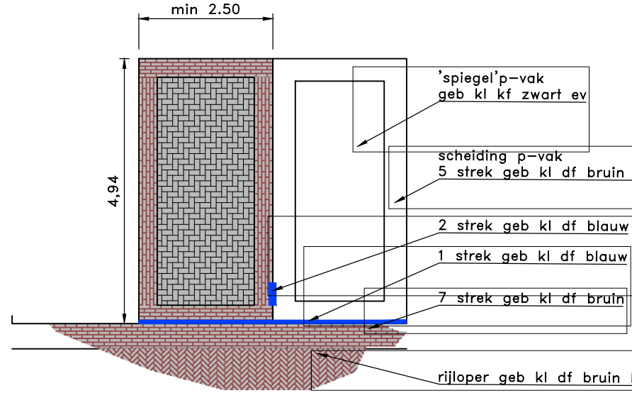
Detail parkeervak 2: conform straatbeeld (II)
