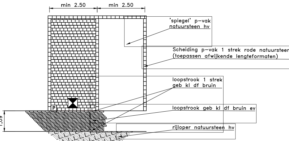
Detail parkeervak 3: natuurkeien (III)
