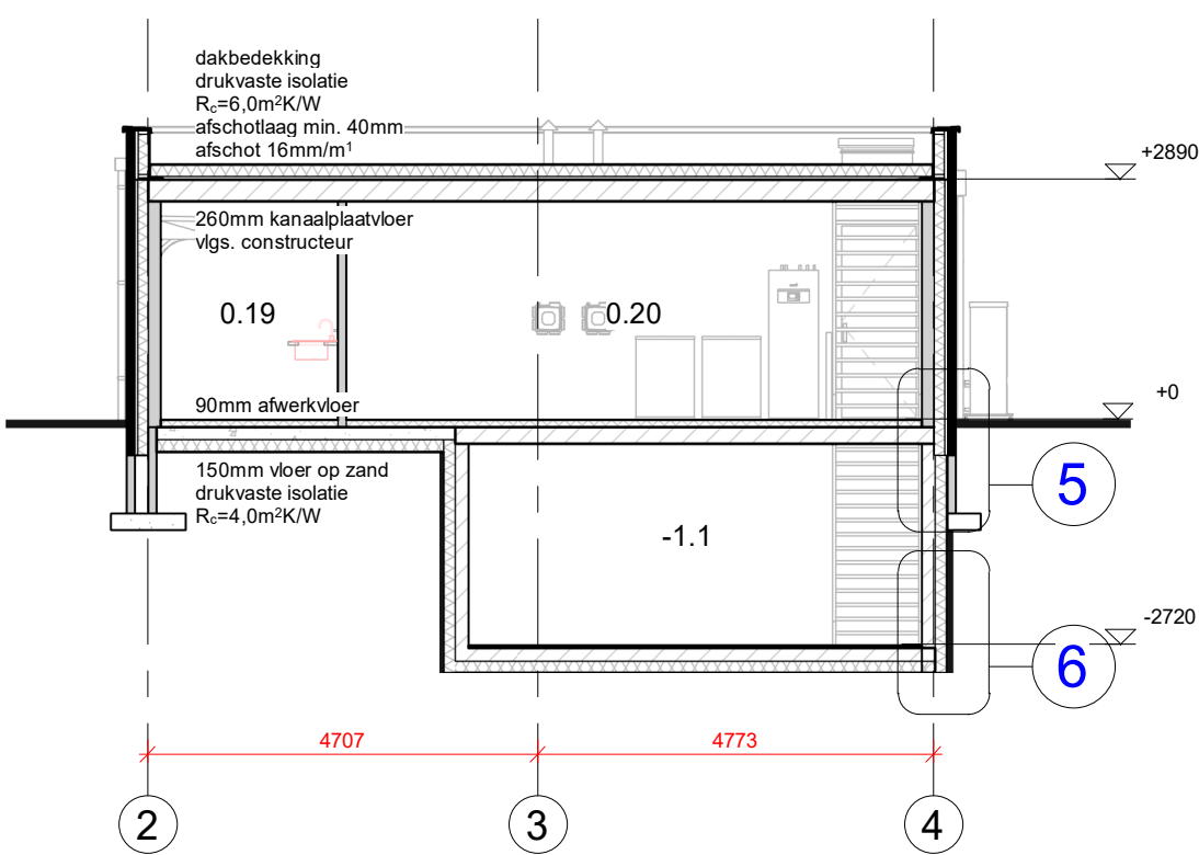
doorsnede C
