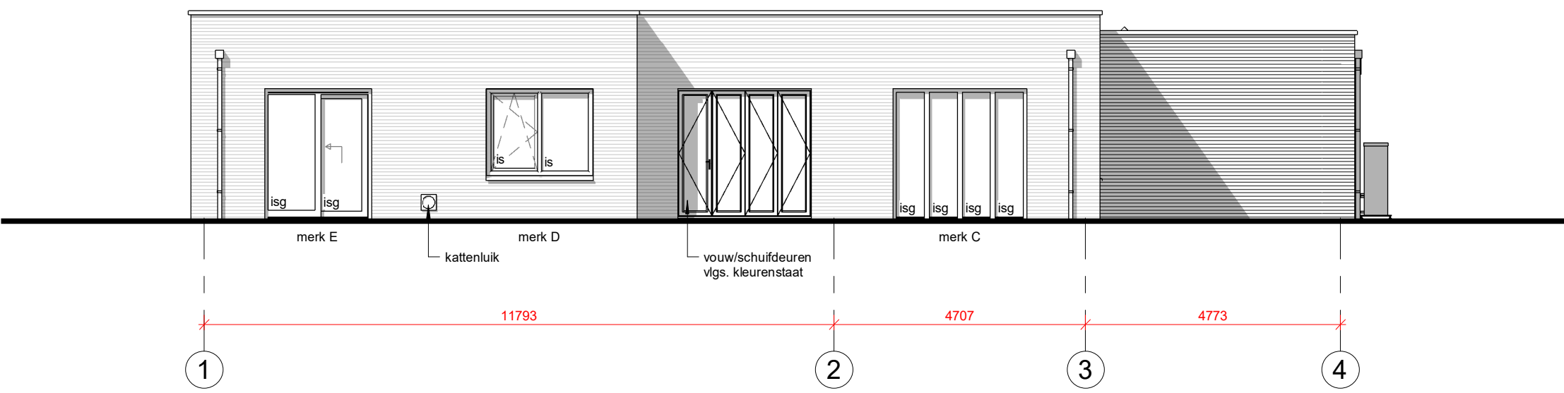
rechter zijgevel
