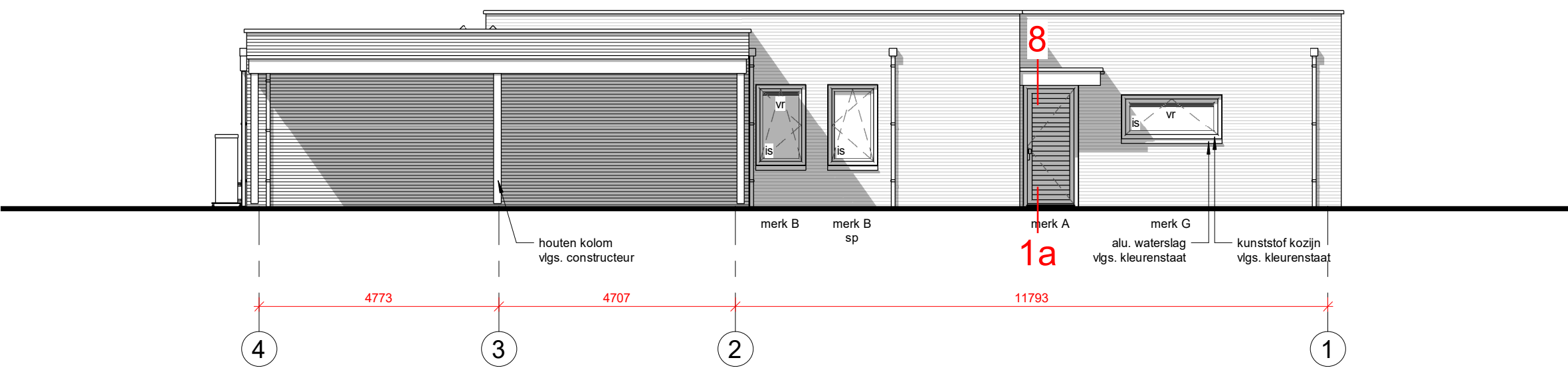
linker zijgevel
