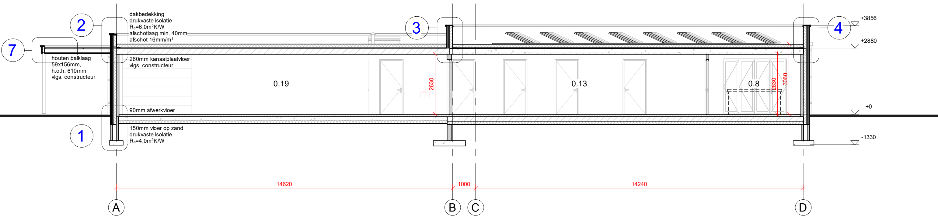
doorsnede A
