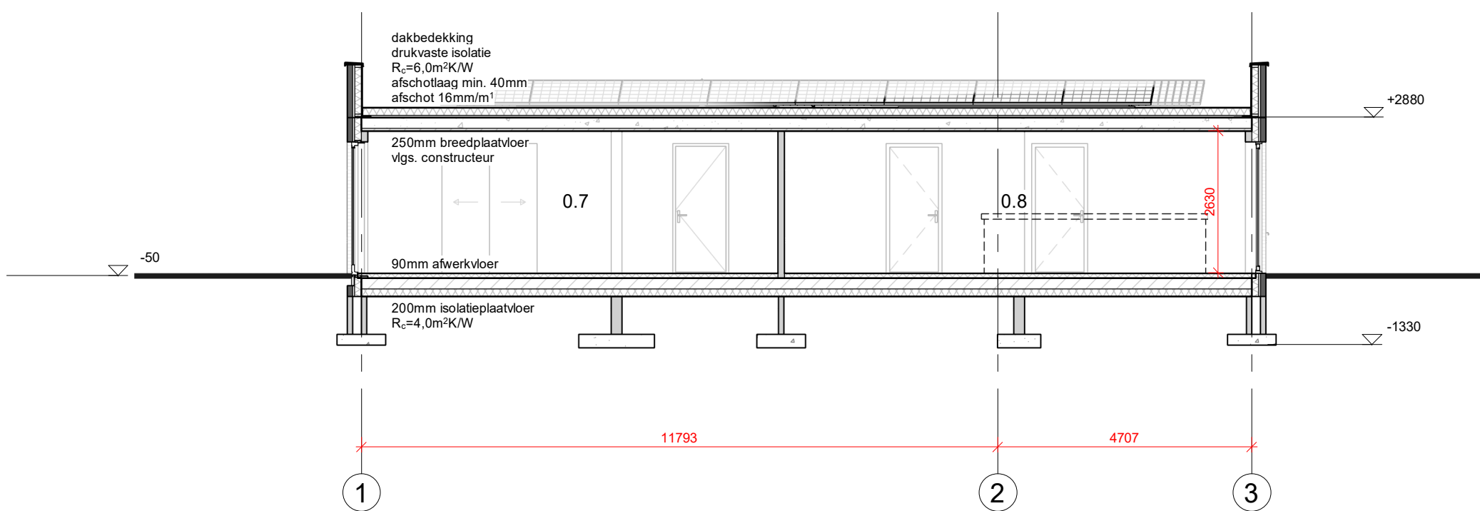
doorsnede B
