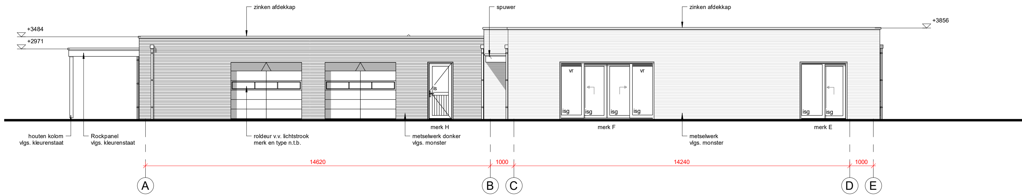
voorgevel
