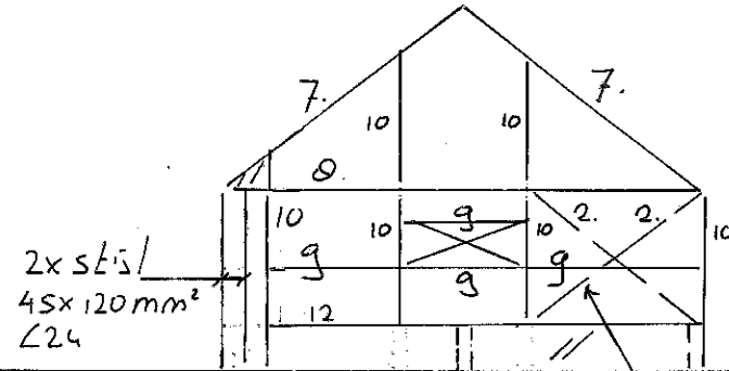
Zijgevel
