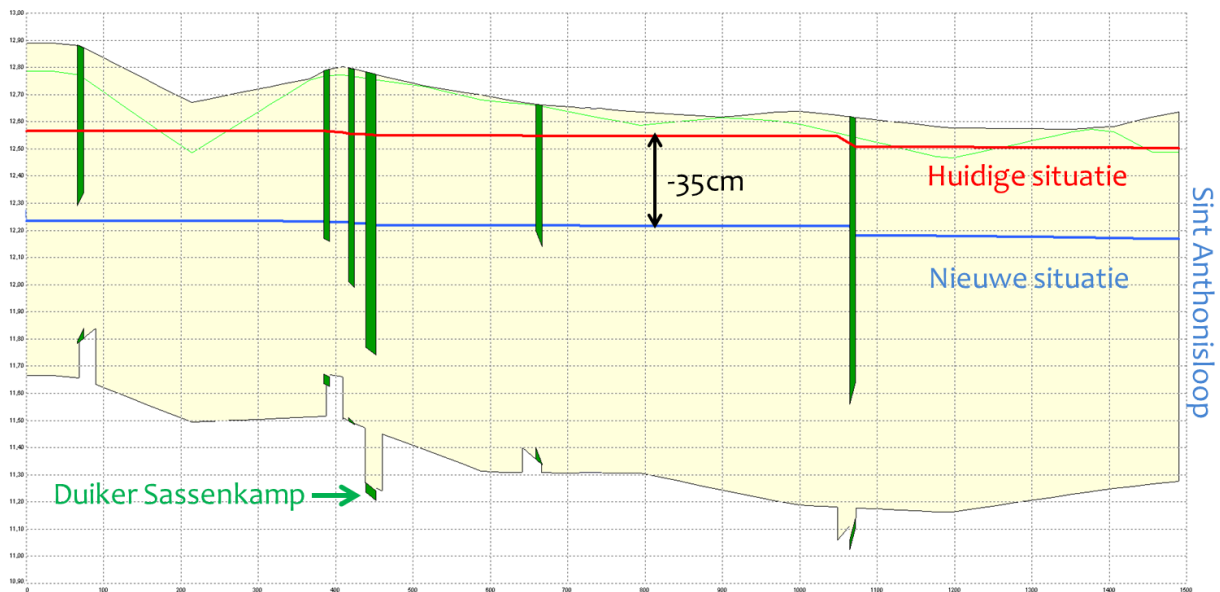
Figuur 6: Verandering waterstand waterloop 108053 (rode lijn = huidige situatie, blauwe lijn = nieuwe situatie)
