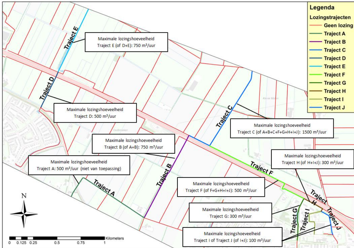
Figuur B1.1: Maximaal toegestane debieten per lozingstraject (aanvulling / gebaseerd op figuur 3.1 in monitorings- en lozingenadvies)
