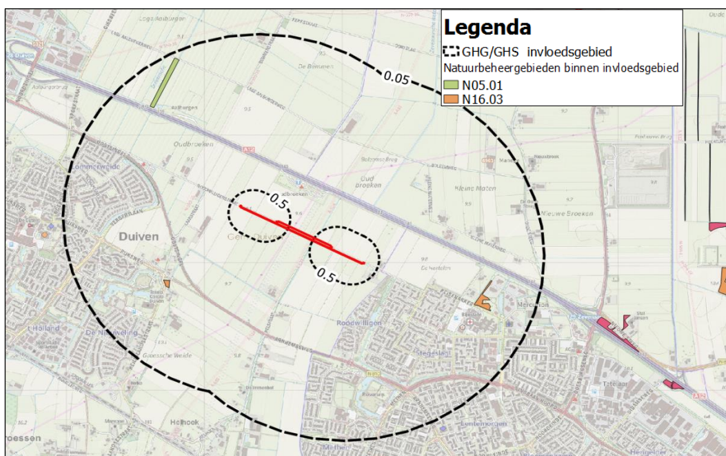
Invoelingsgebied (gemiddeld hoogste grondwaterstand) bronbemaling langs de Roodwilligenstraat, met natuurbeheertypen
