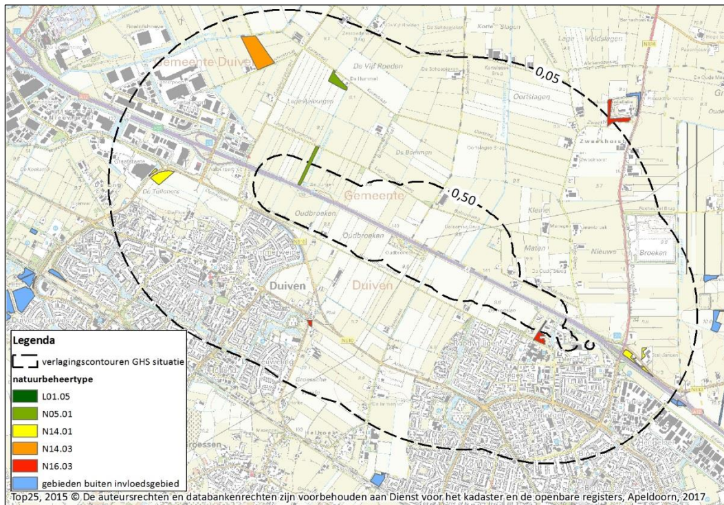
Invoelingsgebied (gemiddeld hoogste grondwaterstand) bronbemaling langs de A12, met natuurbeheertypen
