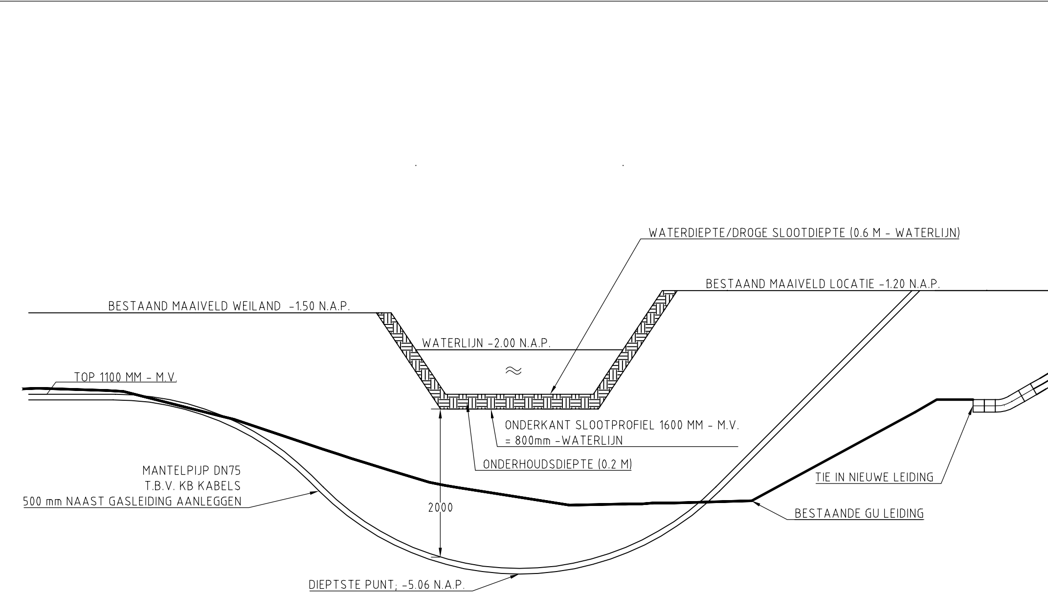
DOORSNEDE A-A
