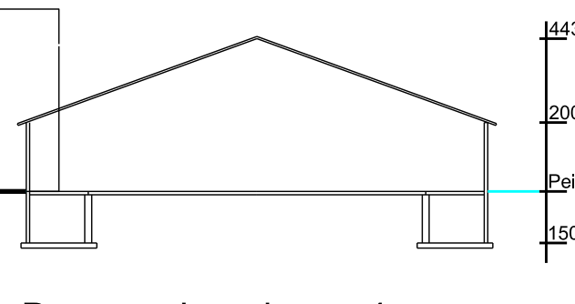
Doorsnede gebouw 4
