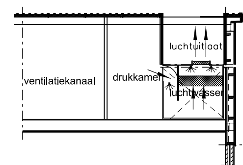
Doorsnede gebouw 9 t.p.v. de wasser
