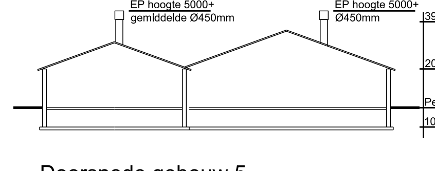
Doorsnede gebouw 5
