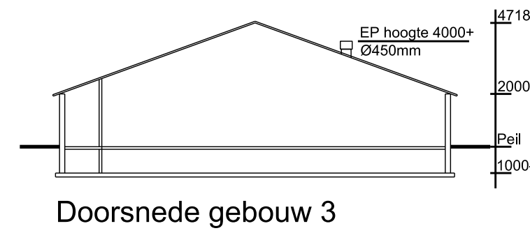
Doorsnede gebouw 3
