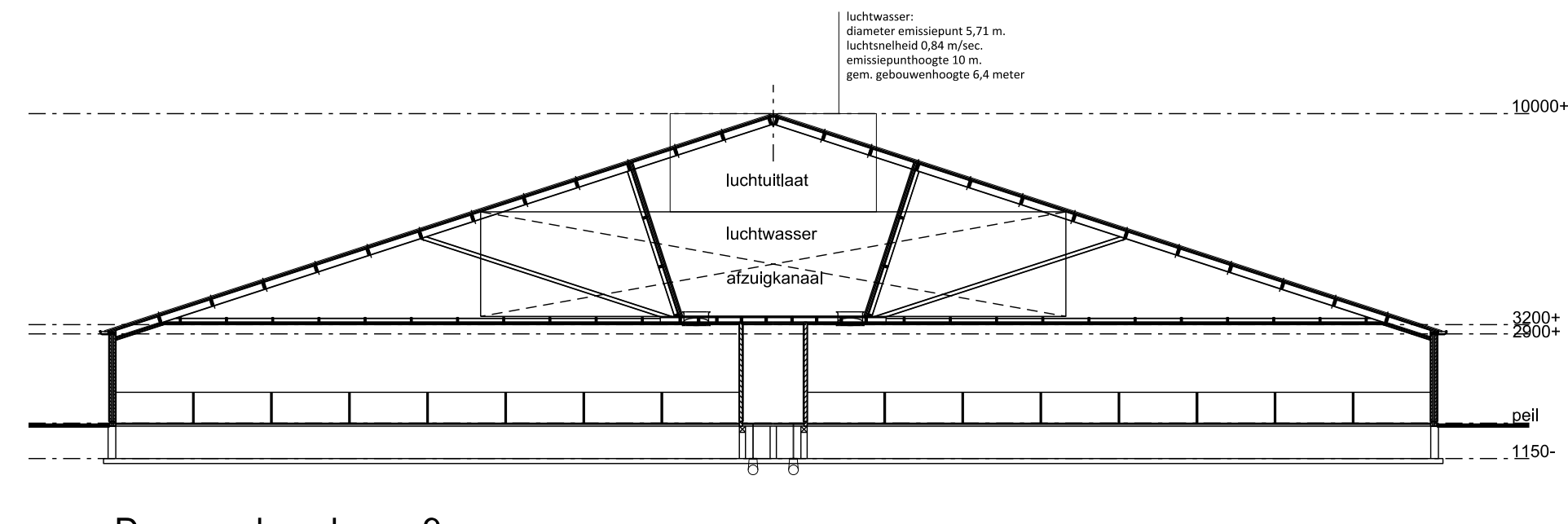
Doorsnede gebouw 9
