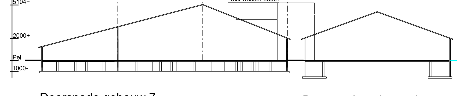
Doorsnede gebouw 7
