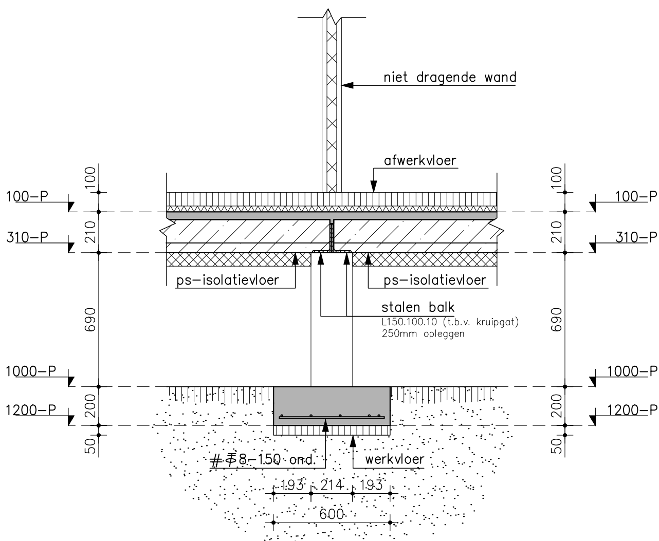
principe kruipgat
