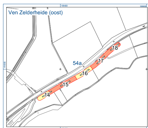
Bijlage 1. Puttenplan.
