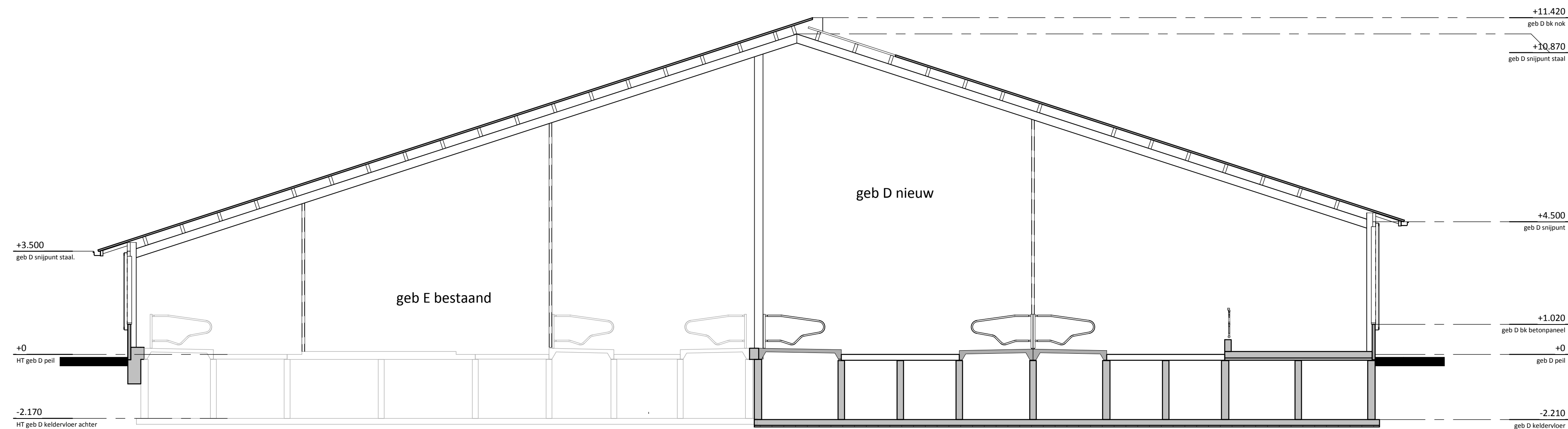
doorsnede DE1
