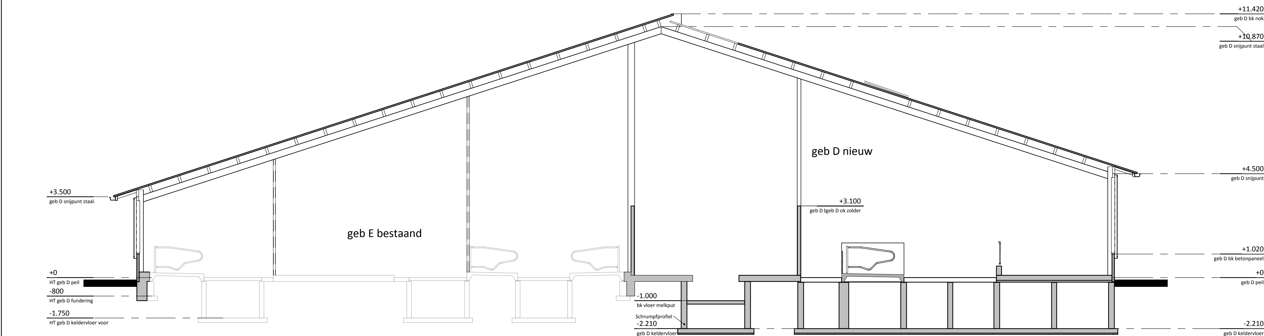
doorsnede DE
