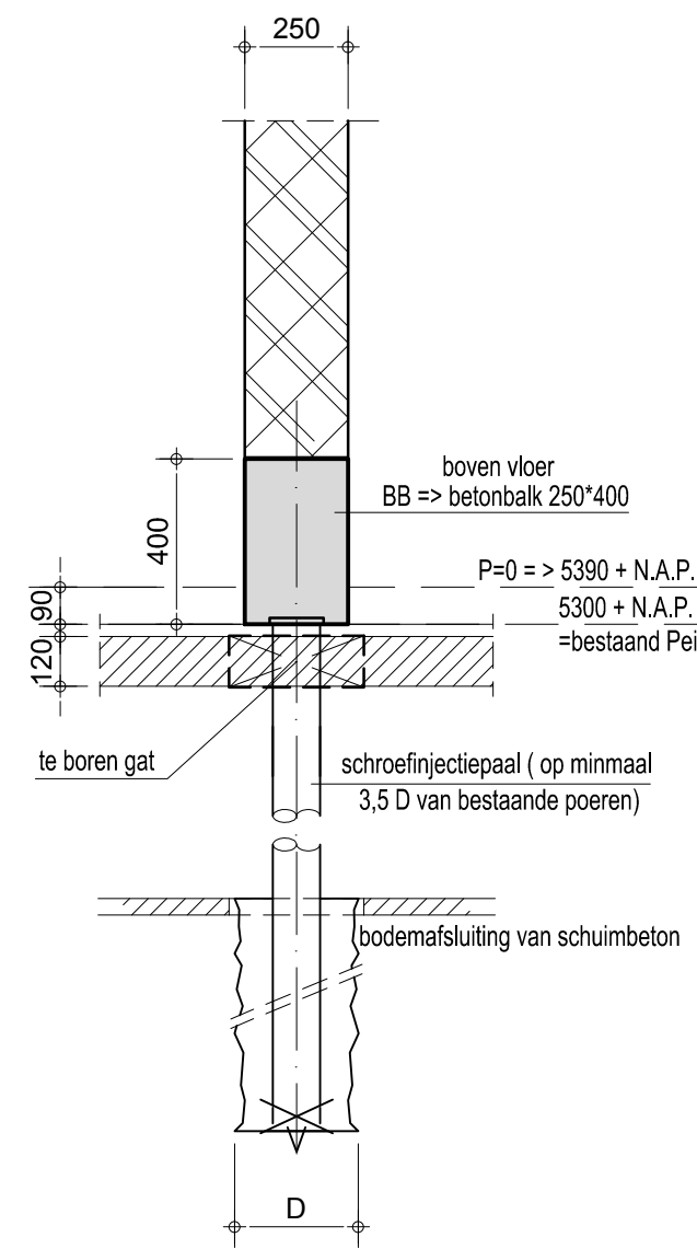
-PRINCIPE- fundatie onder nieuwe bouwmuur
