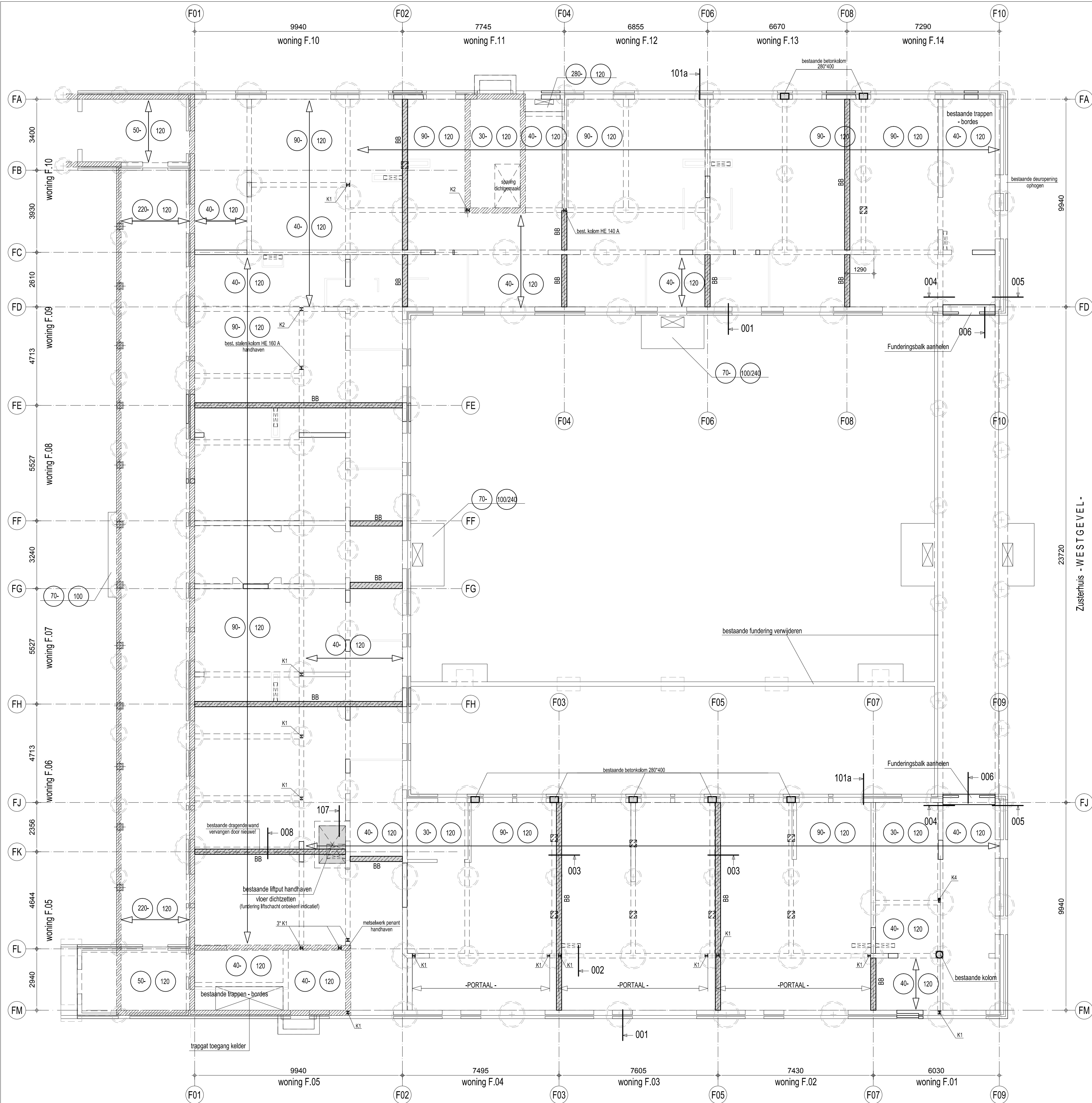
-PRINCIPE- fundatie onder nieuwe bouwmuur
