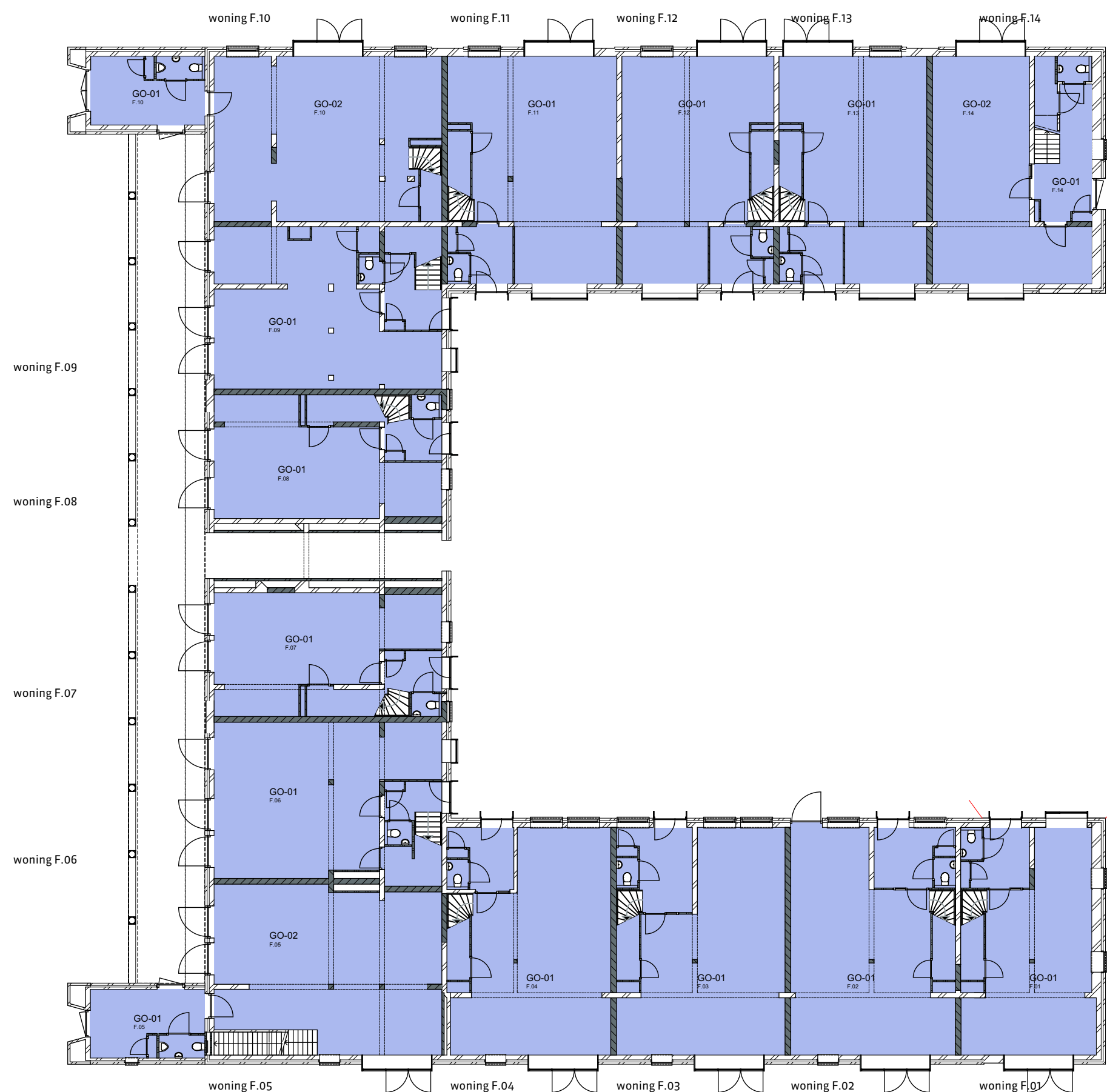
begane grond
