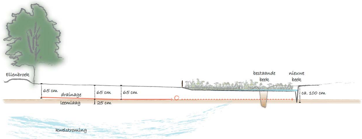
Figuur 3-6 Profiel ter hoogte van Vessem.
