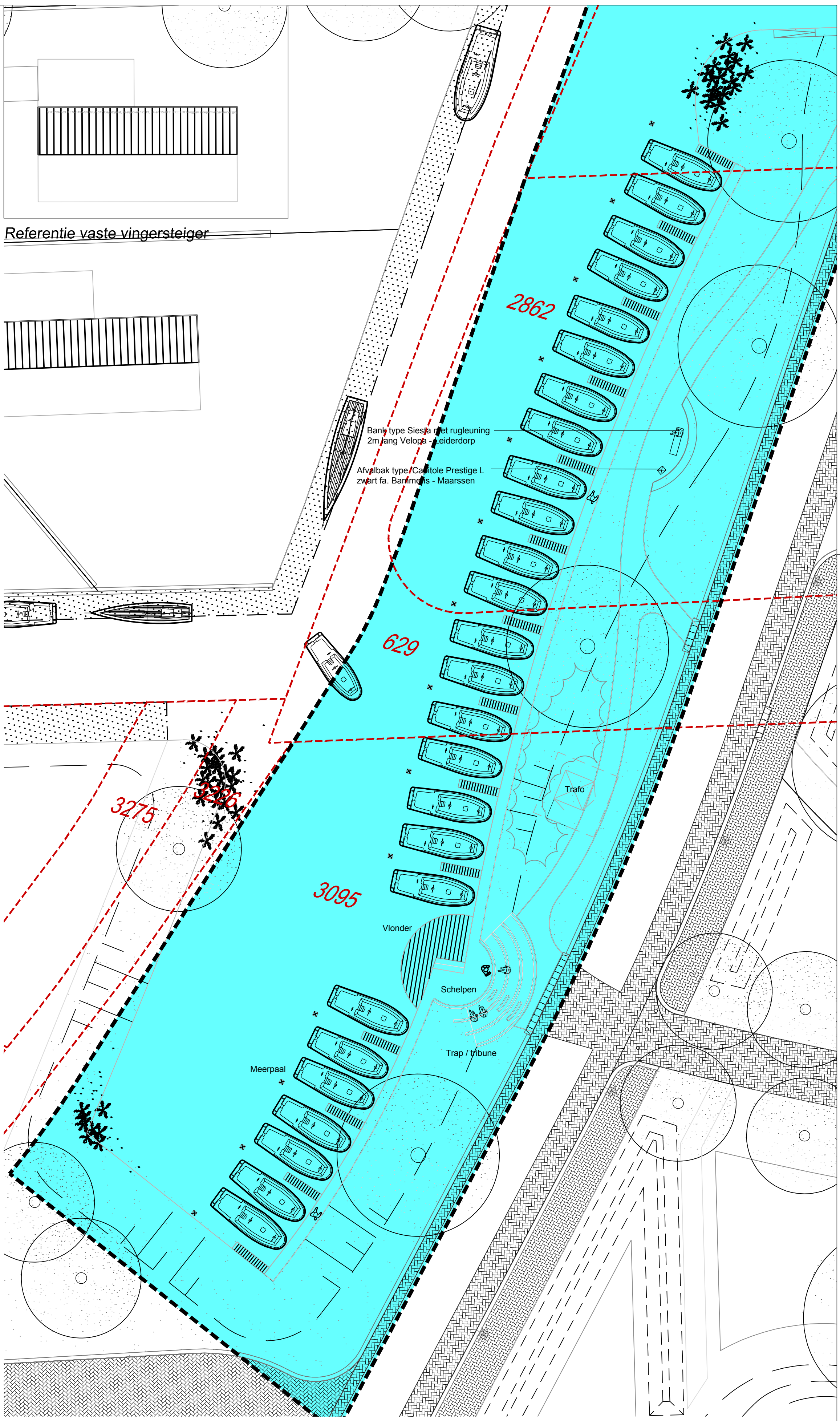
Aanlegsteigers Binnenrijn t.h.v. Landskroonpark - schaal 1:200
