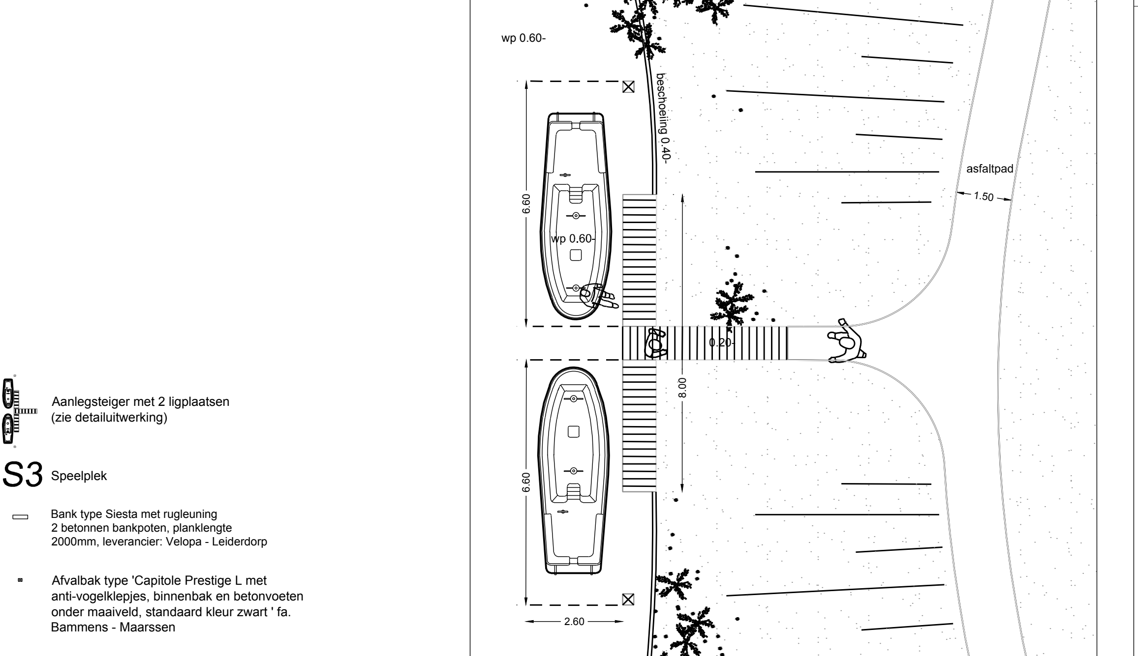
Uitwerking aanlegsteiger - schaal 1:100
