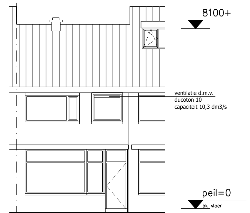
Voorgevel nieuw
