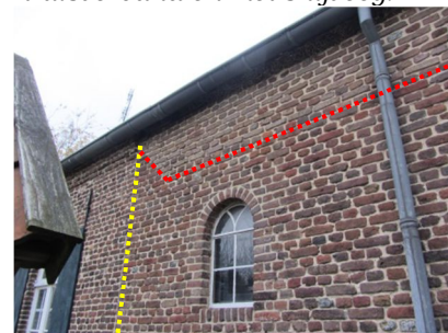
Afb. 7 Lijnen in het metselwerk: links wildverband uit 1920, rechts kruisverband in twee soorten baksteen uit 1744.
