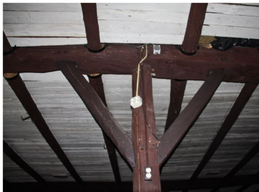
Afb. 47 Detail van een van de staanders met moerbalken en schoren.
