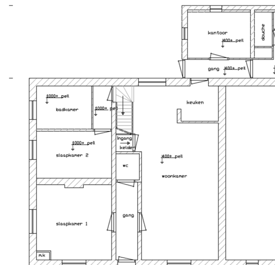
Afb. 55 Plattegrond van de begane grond
