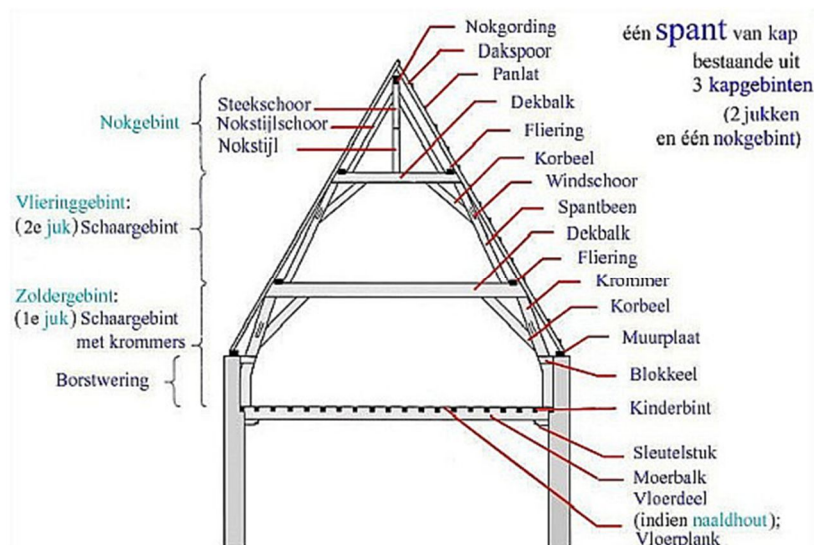
Afb. 37 Schematische weergave van een soortgelijke kap als Kasteellaan 1 (bron: www.joostdevree.nl )
