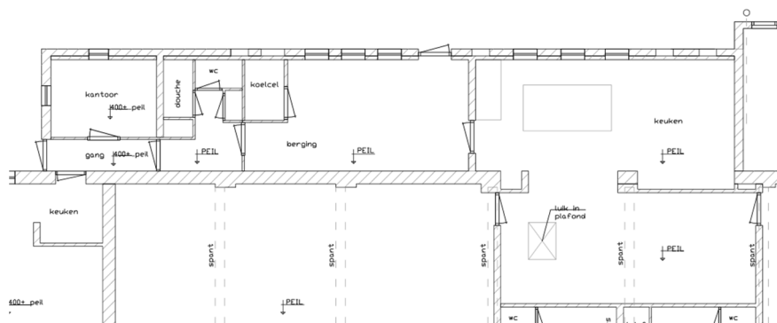
Afb. 67 Plattegrond van het stalvolume.
