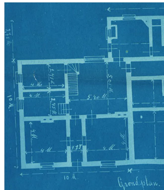
Afb. 105 Nieuwe situatie woonhuis, 1920 (G.A.H. inv.nr 3674)
