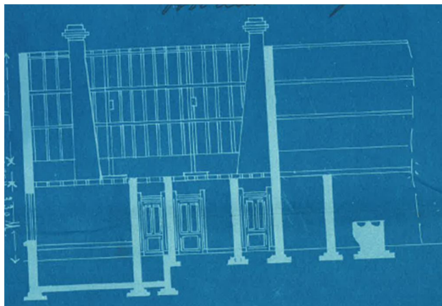
Afb. 106 Nieuwe situatie woonhuis, 1920. Oost-west doorsnede (G.A.H. inv.nr 3674)
