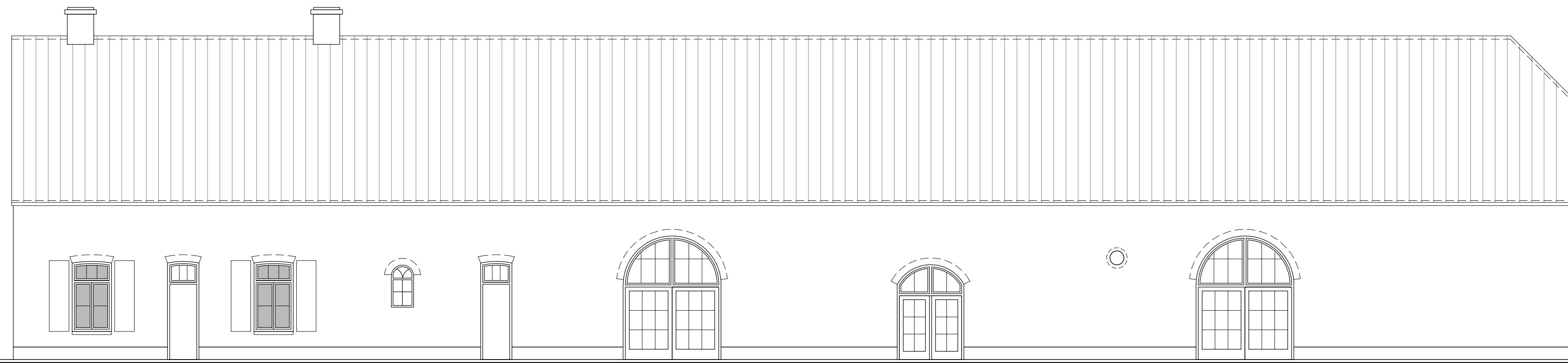
- NOORDGEVEL -
