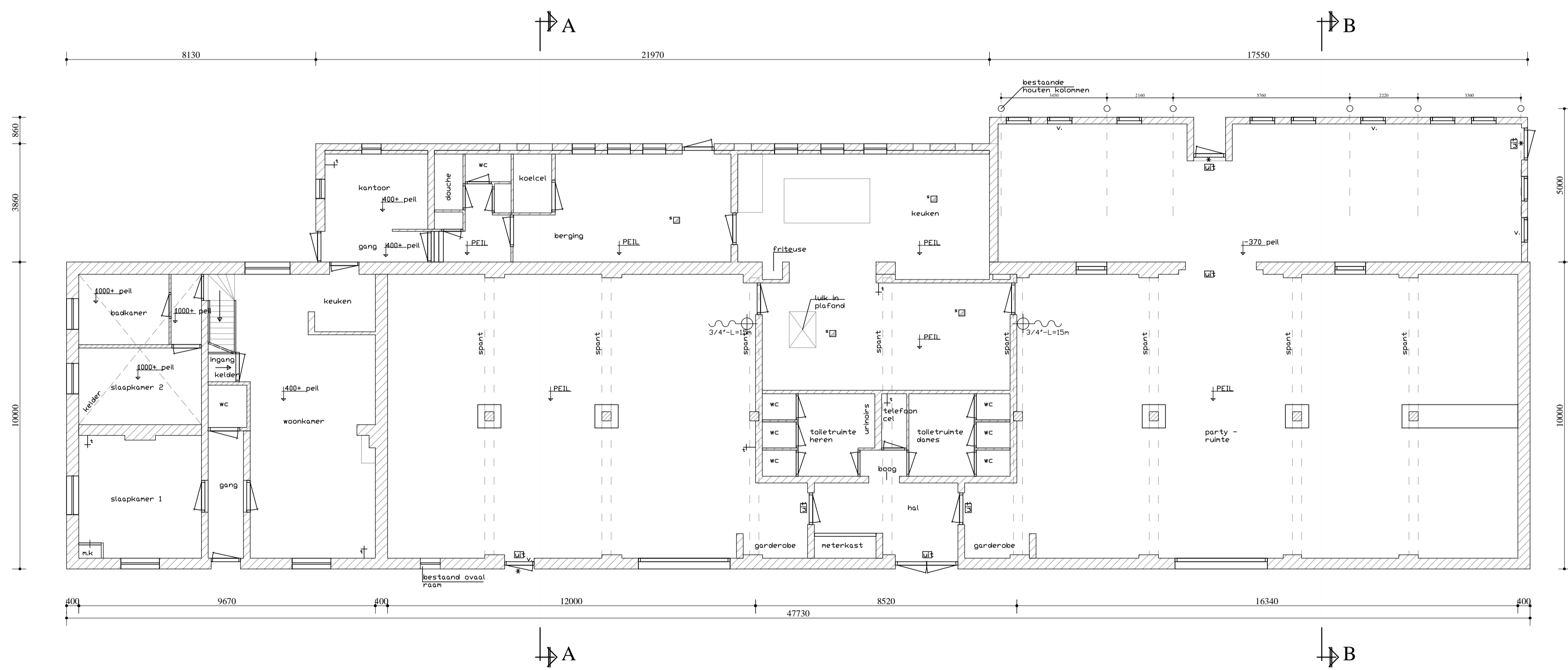
- BEGANE GROND -
