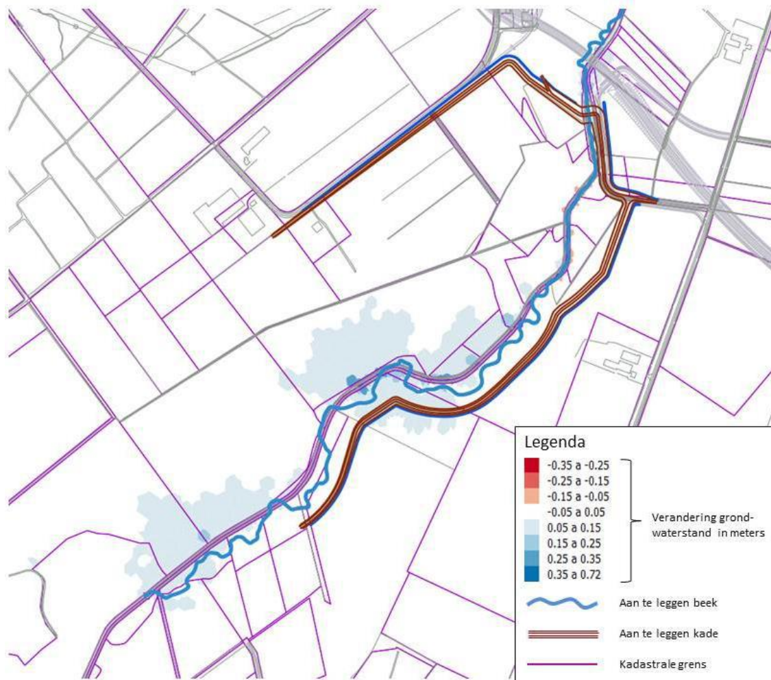
Figuur 39 Effecten grondwater, gemiddelde hoogste grondwaterstand (GLG)
