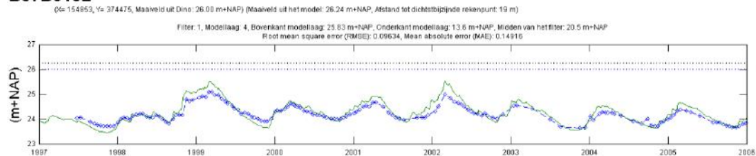
Figuur 20 Vergelijking meting (blauw) en berekening (groen) bij peilbuis B57B0152.
