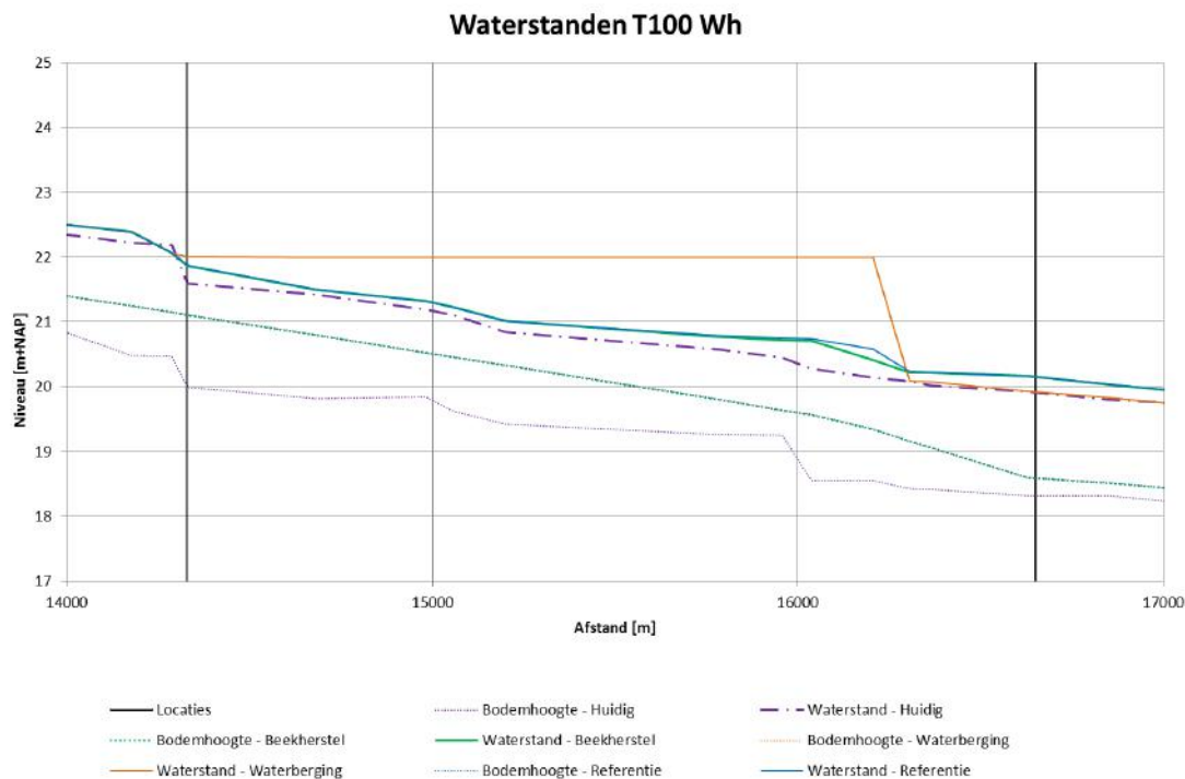
Figuur 4-5 Lengteprofiel berekende waterstanden T100Wh waterbergingsgebied
