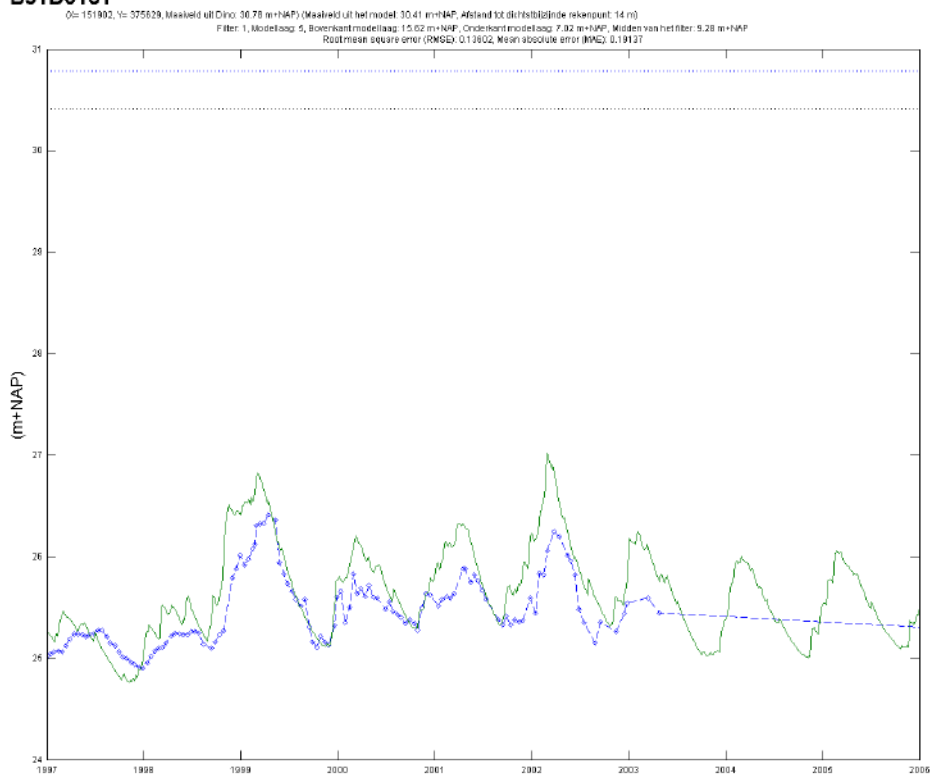
Figuur 19 Vergelijking meting (blauw) en berekening (groen) bij peilbuis B51D0131.
