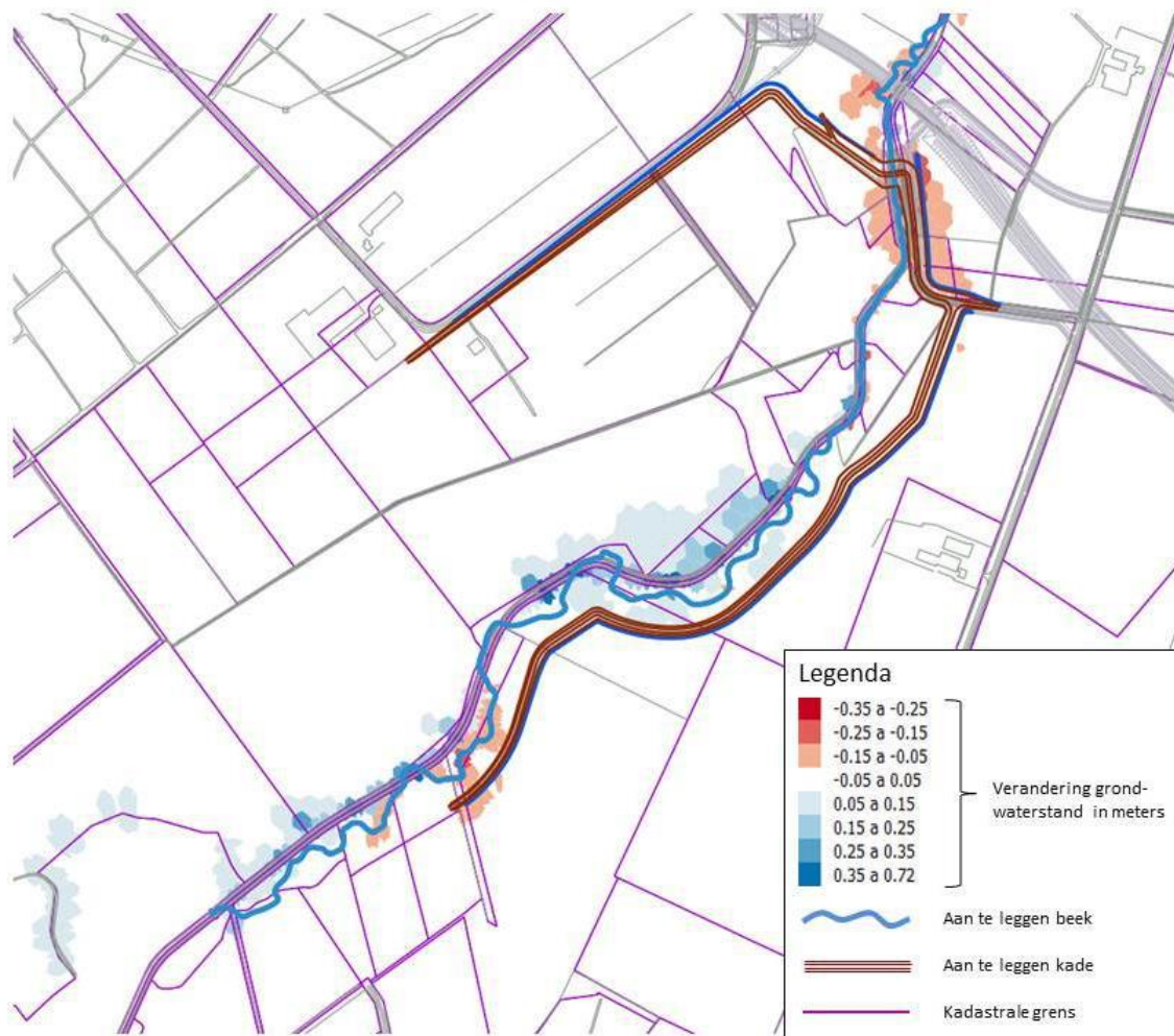
Figuur 37 Effecten grondwater, gemiddelde hoogste grondwaterstand (GHG)
