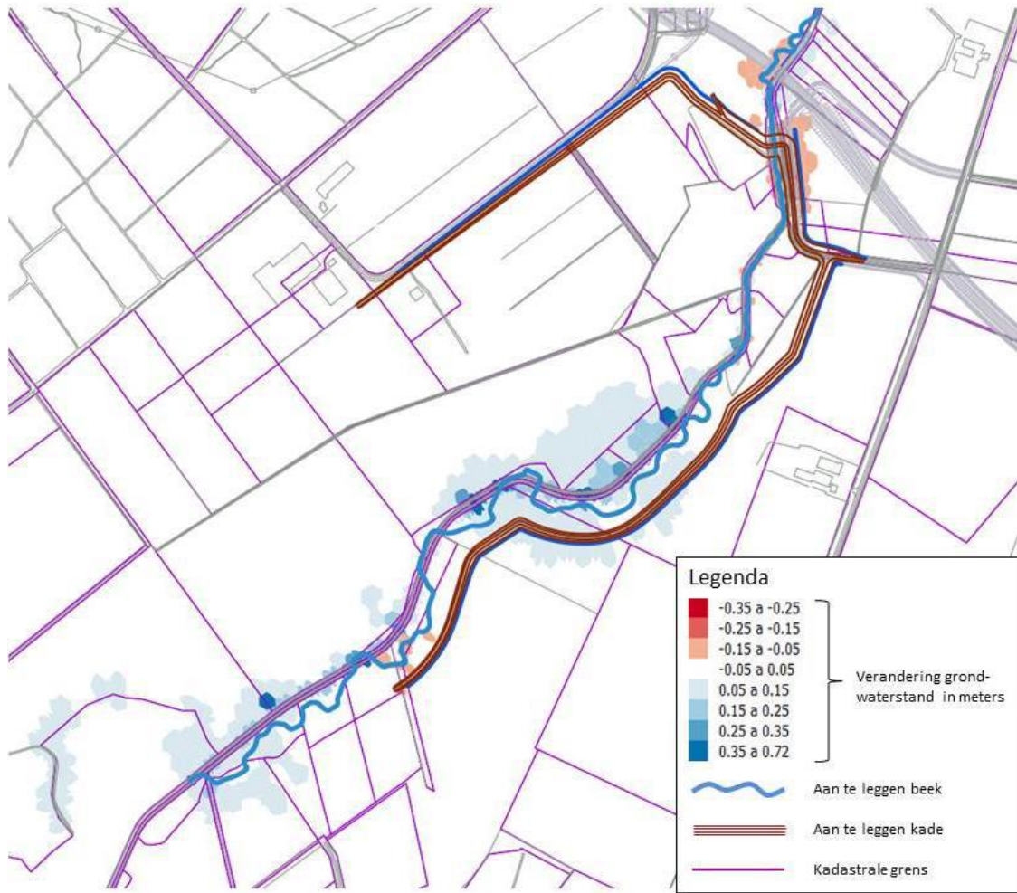
Figuur 38 Effecten grondwater, gemiddelde hoogste grondwaterstand (GVG)
