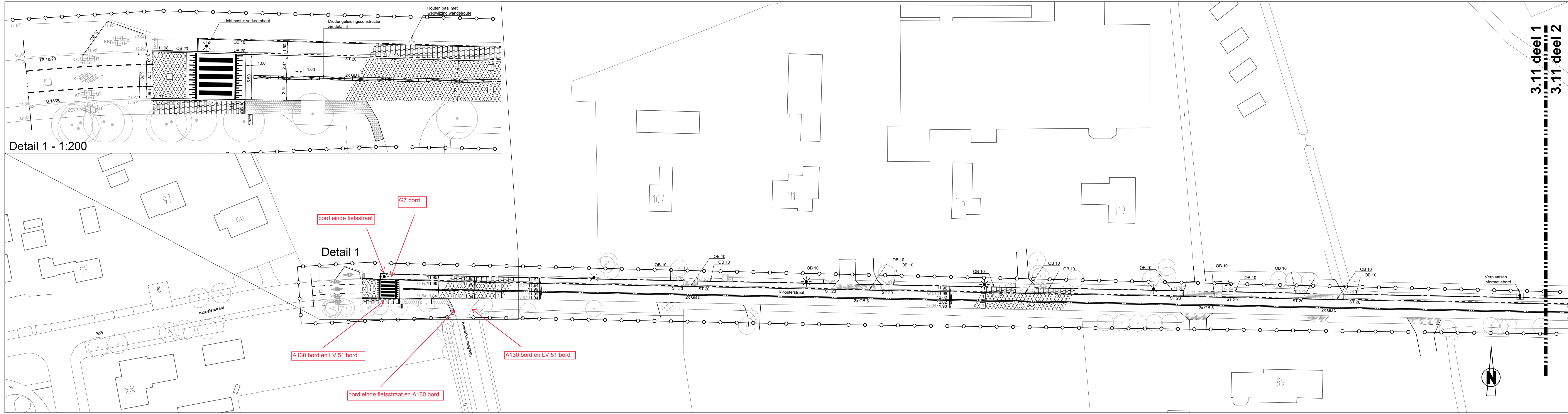
Deel 1 - 1:500
