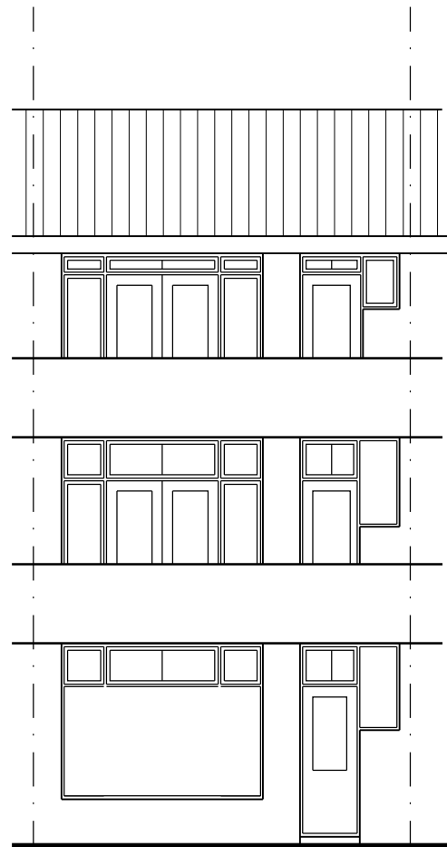
Achtergevel
