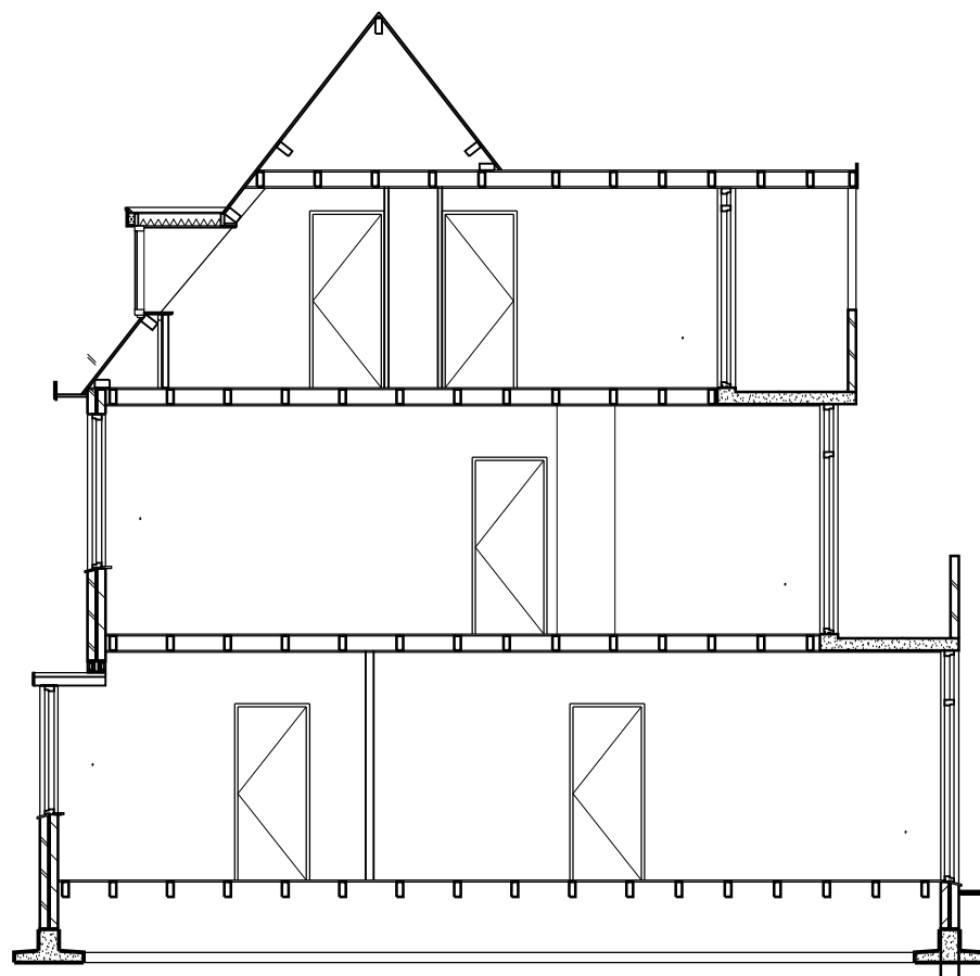
Doorsnede
