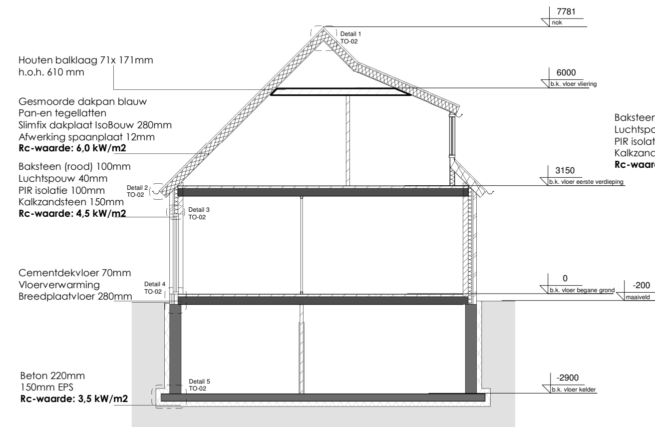
Doorsnede A-A 1 : 100
