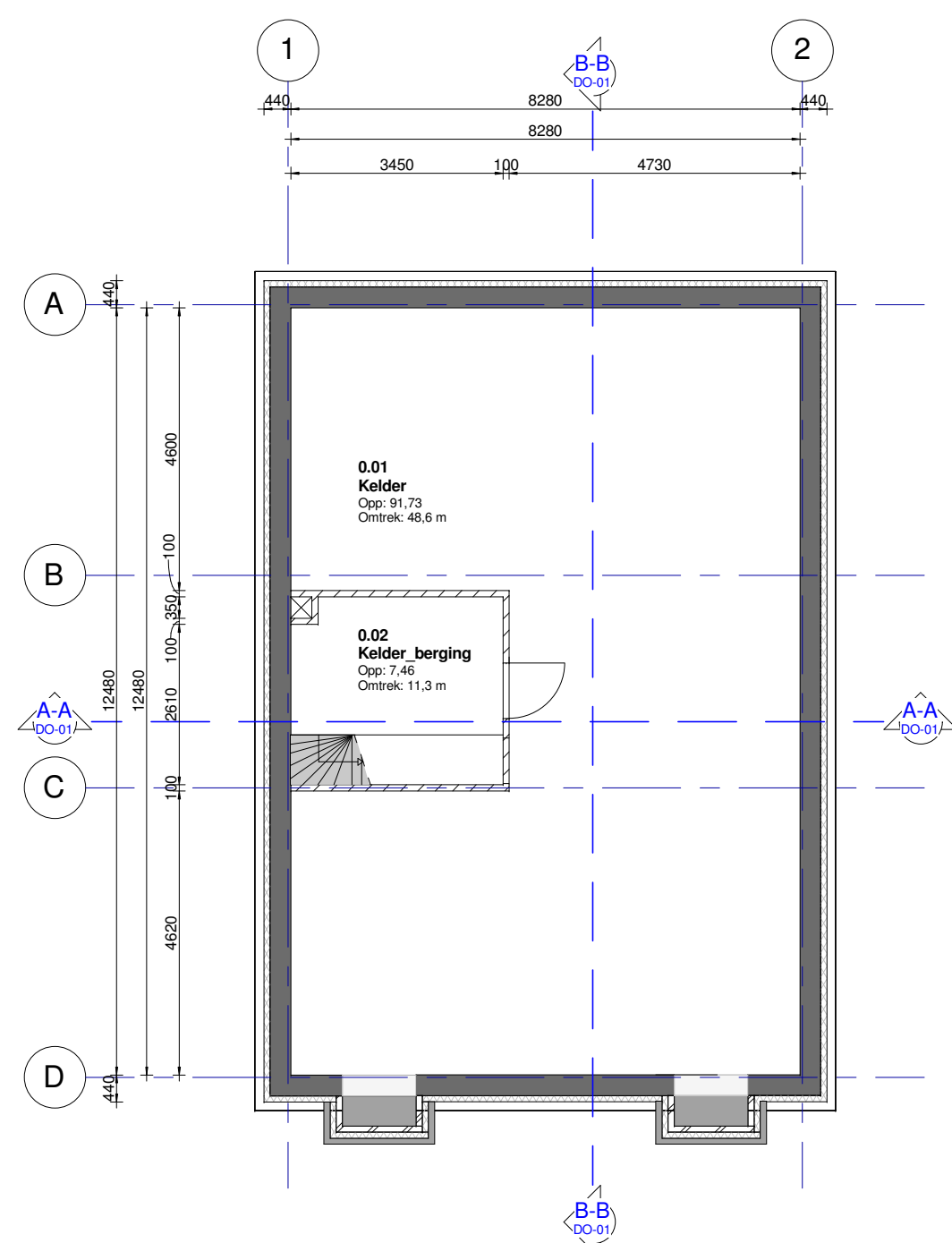
Kelder 1 : 100
