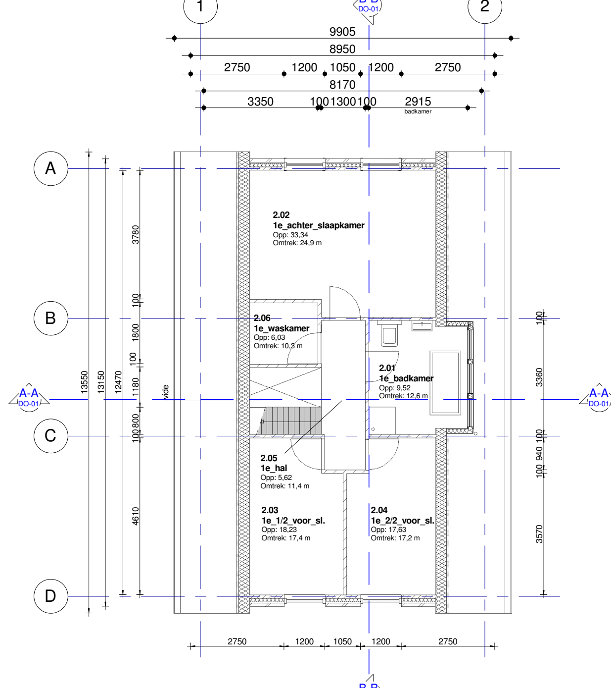
Verdieping 1 1 : 100
