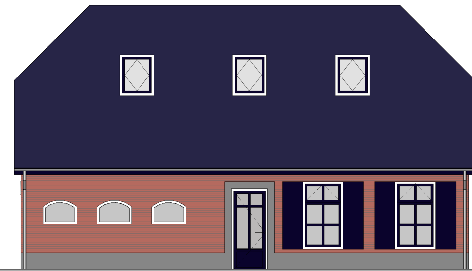
Voorgevel 1 : 100
