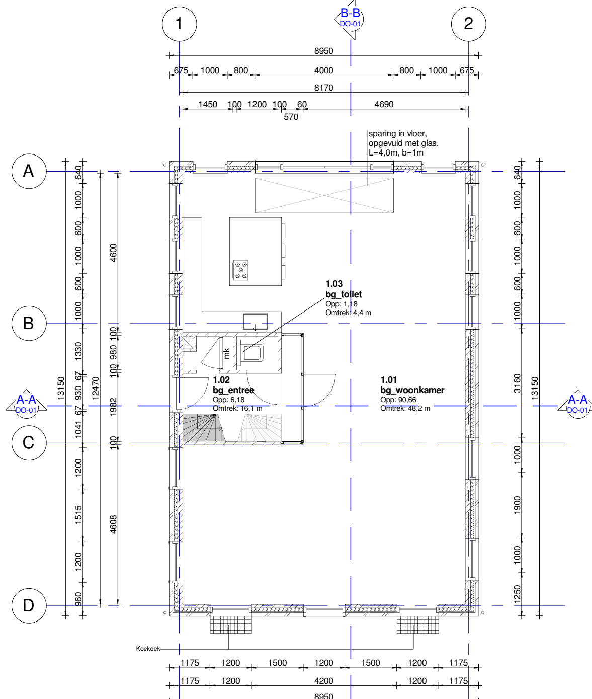
Begane grond 1 : 100
