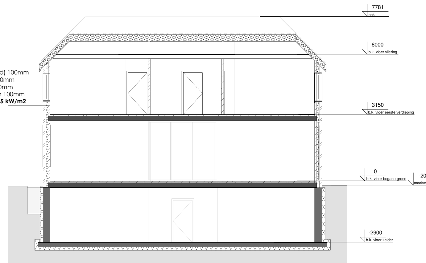
Doorsnede B-B 1 : 100
