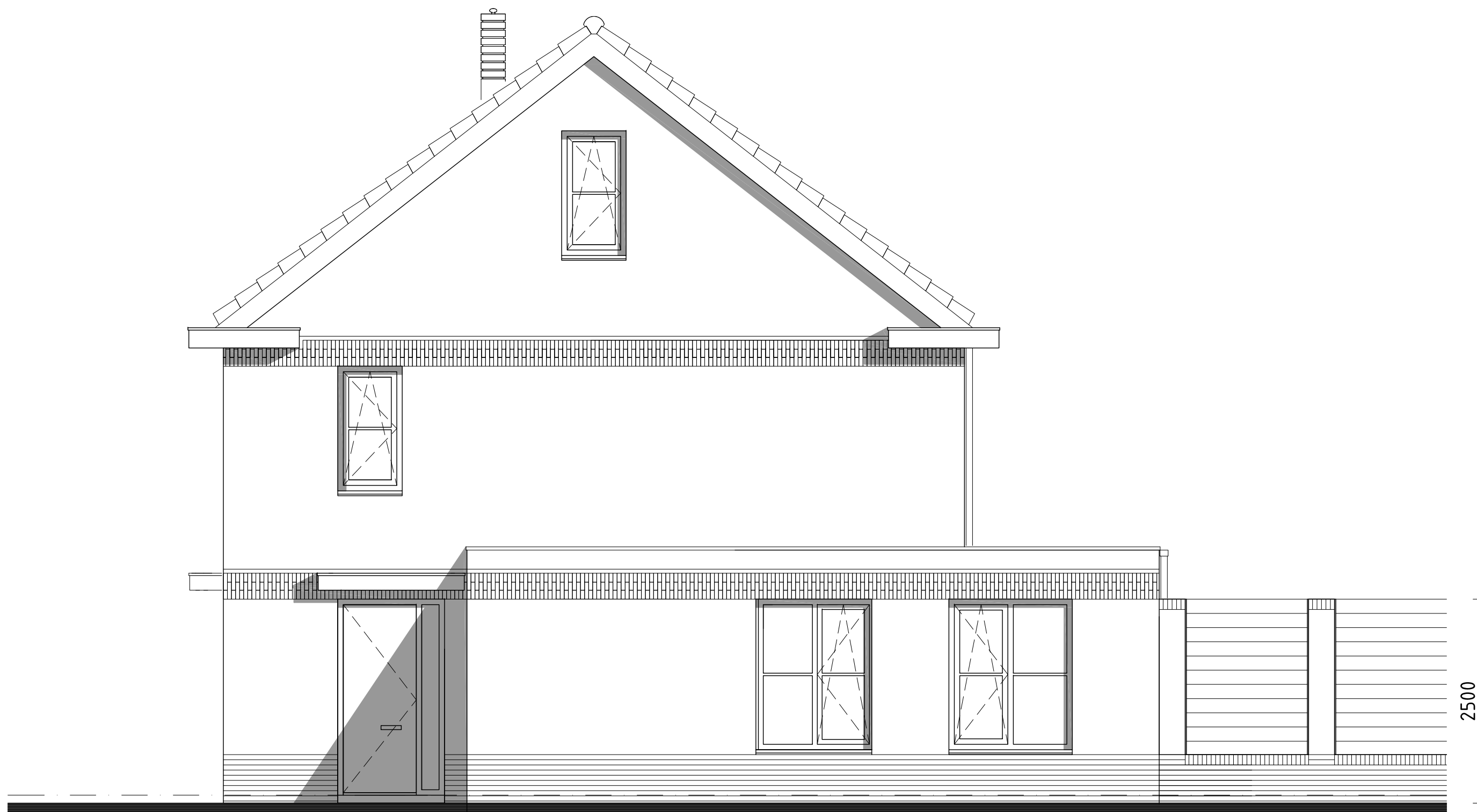
rechter zijgevel
