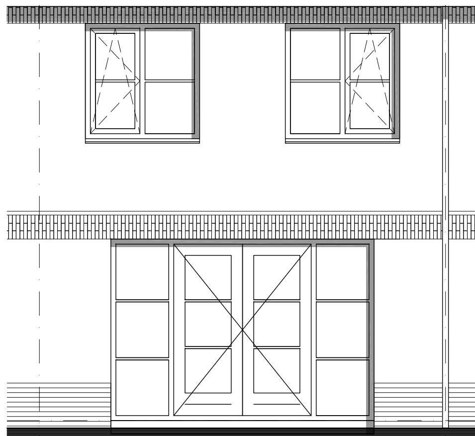
achtergevel
