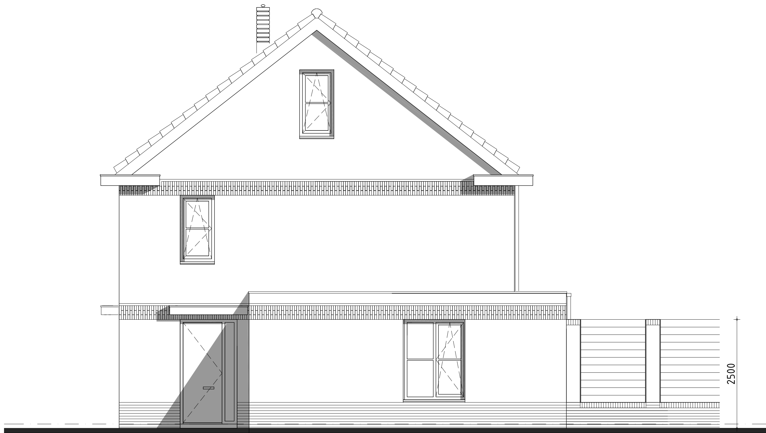
rechter zijgevel
